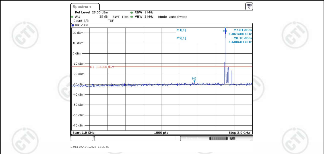
Band25-20MHz-QPSK-26140-1RB#0-Range2:1000~2000MHz
