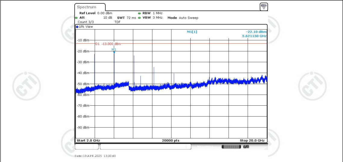
Band25-20MHz-QPSK-26365-1RB#0-Range3:2000~20000MHz
