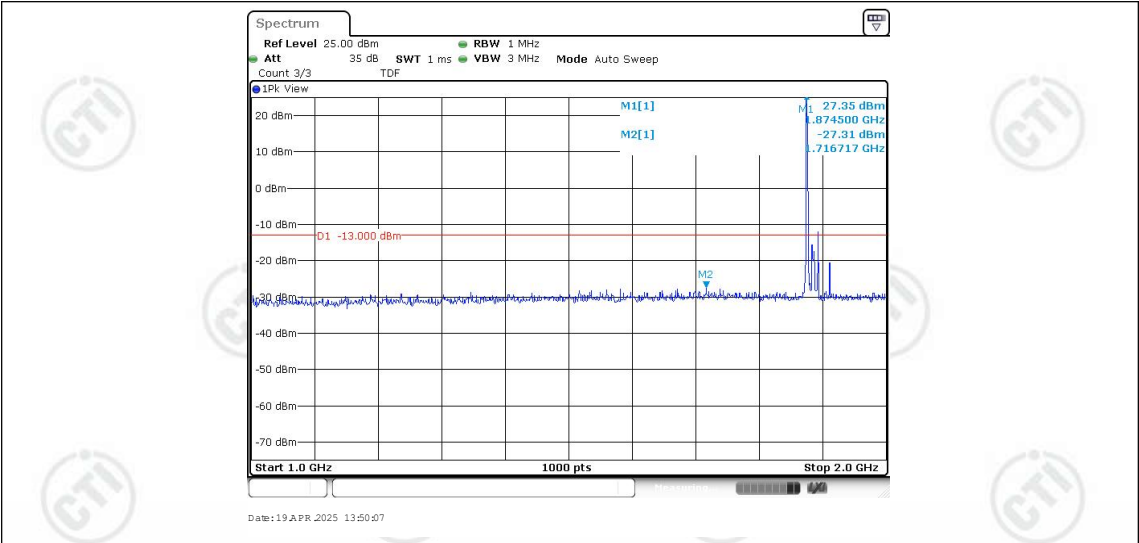
Band25-20MHz-16QAM-26365-1RB#0-Range2:1000~2000MHz
