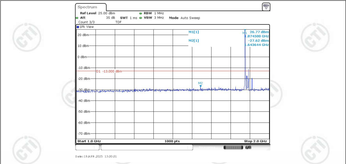
Band25-20MHz-QPSK-26365-1RB#0-Range2:1000~2000MHz
