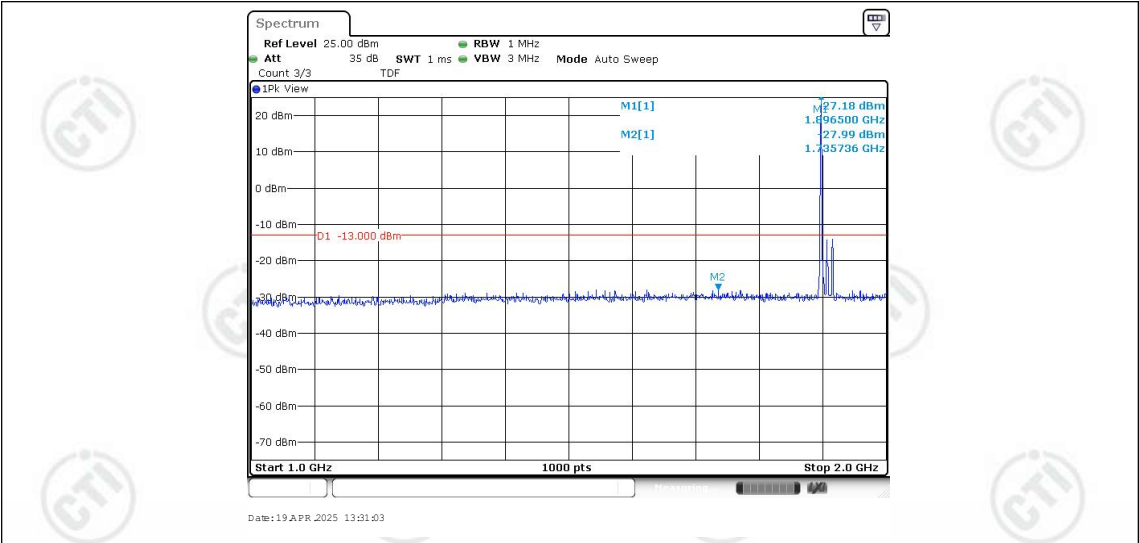
Band25-20MHz-QPSK-26590-1RB#0-Range2:1000~2000MHz
