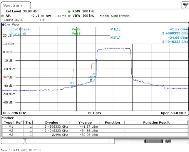
Band41-10MHz-QPSK-39700-50RB#0
