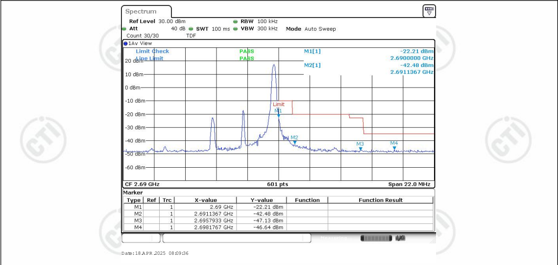
Band41-5MHz-16QAM-41565-1RB#24
