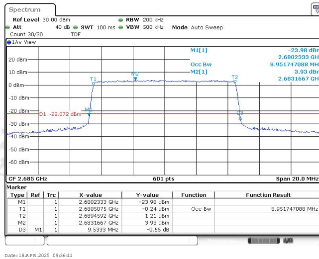
Band41-10MHz-QPSK-41540-50RB#0-8.952
