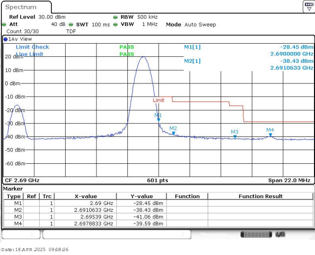
Band41-20MHz-16QAM-41490-1RB#99
