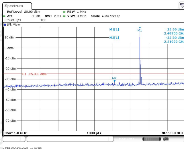
Band41-10MHz-QPSK-39700-1RB#0-Range2:1000~3000MHz
