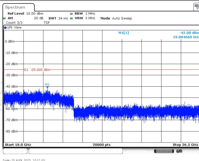
Band41-10MHz-QPSK-39700-1RB#0-Range4:18000~26500MHz
