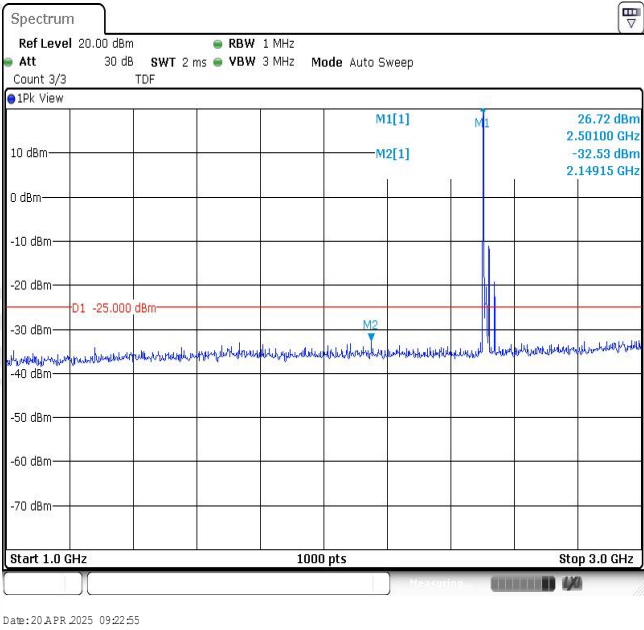
Band7-20MHz-QPSK-20850-1RB#0-Range2:1000~3000MHz
