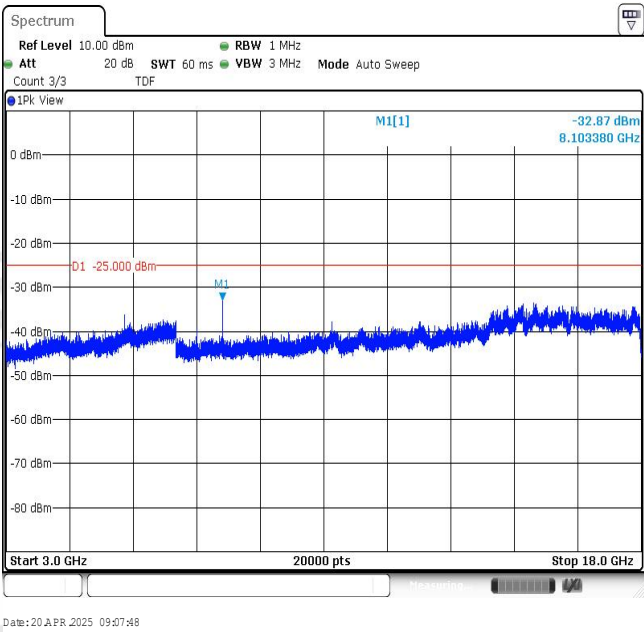
Band7-10MHz-QPSK-20800-1RB#0-Range3:3000~18000MHz
