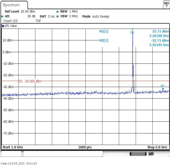
Band7-10MHz-QPSK-21400-1RB#0-Range2:1000~3000MHz
