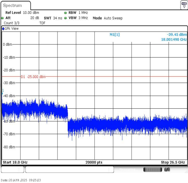
Band7-20MHz-QPSK-21100-1RB#0-Range4:18000~26500MHz
