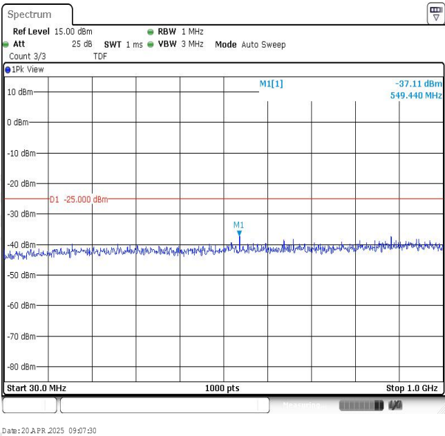
Band7-10MHz-QPSK-20800-1RB#0-Range1:30~1000MHz
