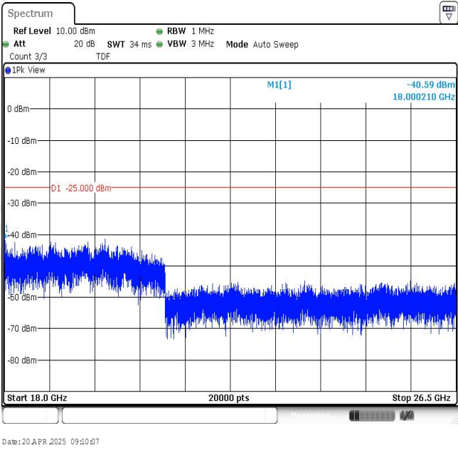
Band7-10MHz-QPSK-21100-1RB#0-Range4:18000~26500MHz
