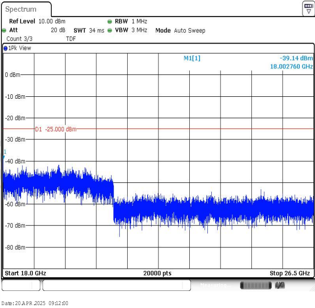
Band7-10MHz-QPSK-21400-1RB#0-Range4:18000~26500MHz
