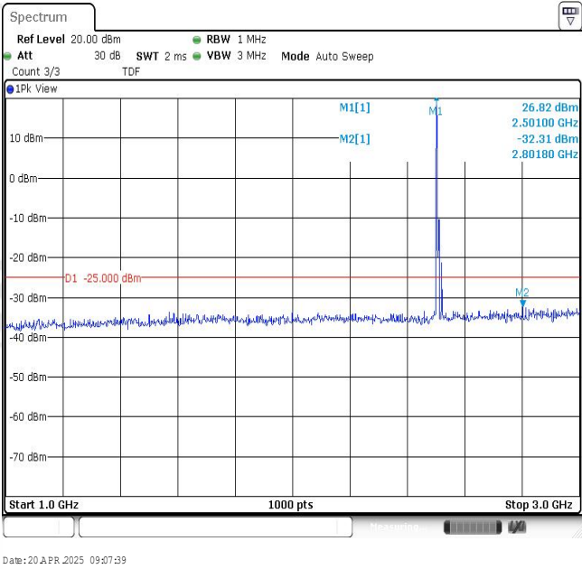
Band7-10MHz-QPSK-20800-1RB#0-Range2:1000~3000MHz
