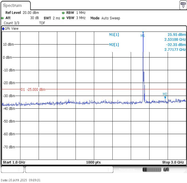
Band7-10MHz-QPSK-21100-1RB#0-Range2:1000~3000MHz
