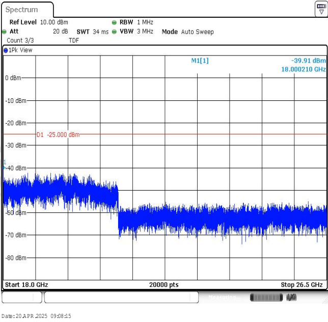
Band7-10MHz-QPSK-20800-1RB#0-Range4:18000~26500MHz
