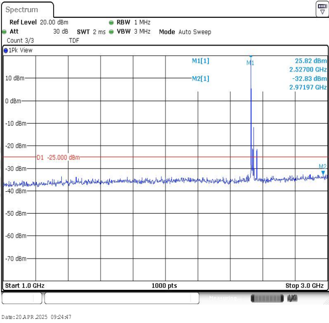
Band7-20MHz-QPSK-21100-1RB#0-Range2:1000~3000MHz
