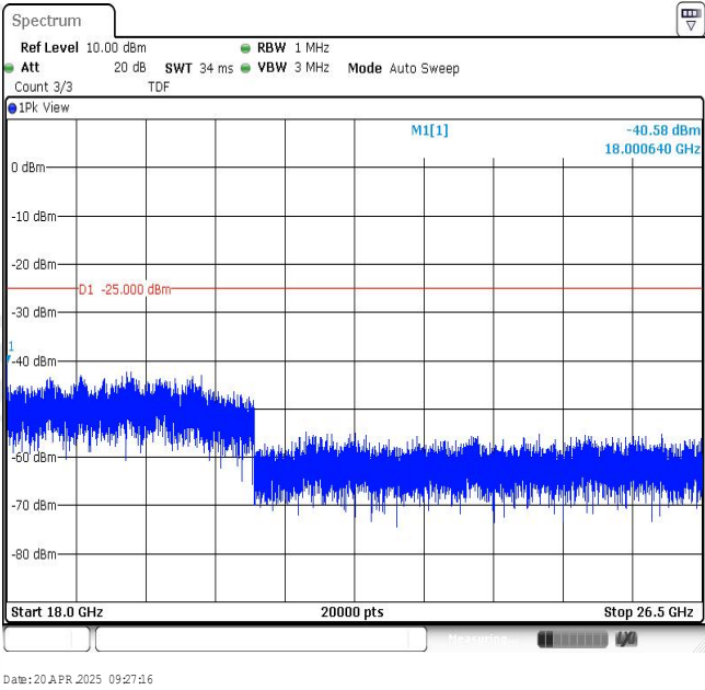
Band7-20MHz-QPSK-21350-1RB#0-Range4:18000~26500MHz
