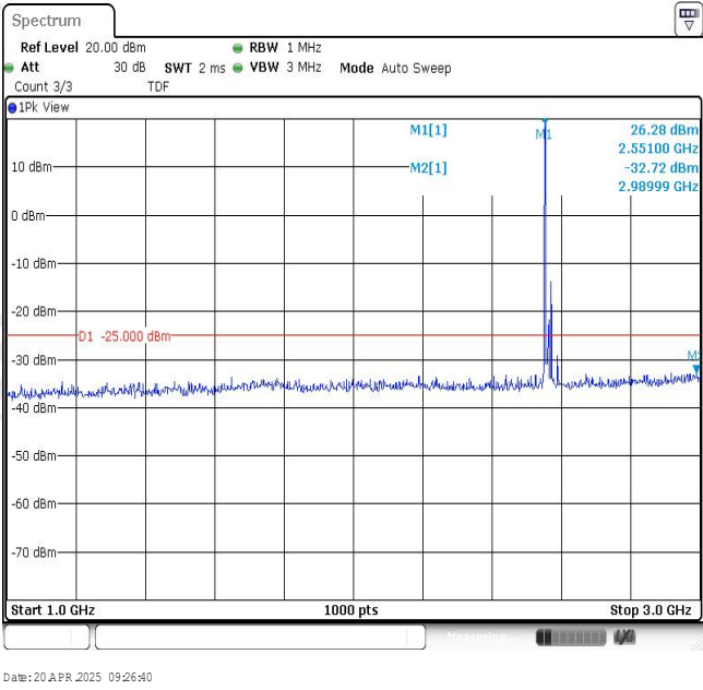
Band7-20MHz-QPSK-21350-1RB#0-Range2:1000~3000MHz
