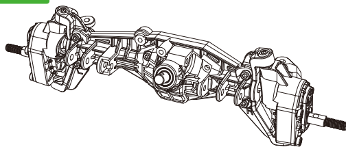
Front Axle Subassembly 前桥组件
