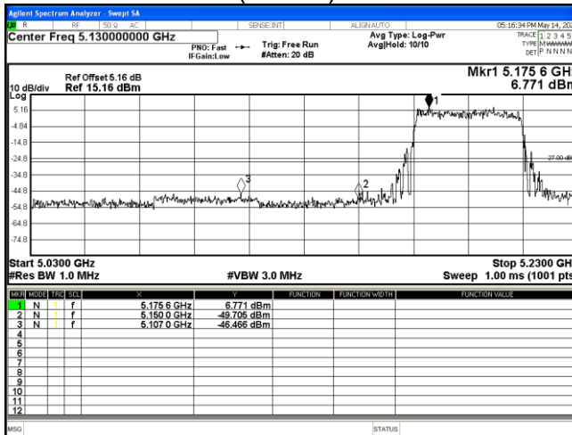
802.11 be(EHT40) 5190MHz
