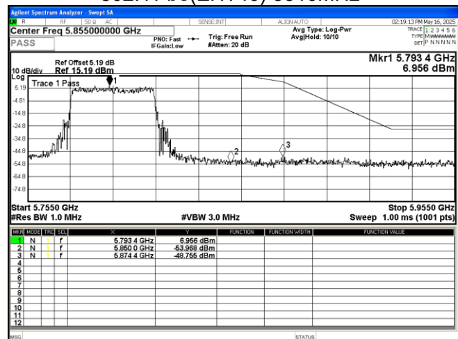
802.11 be(EHT40) 5795MHz
