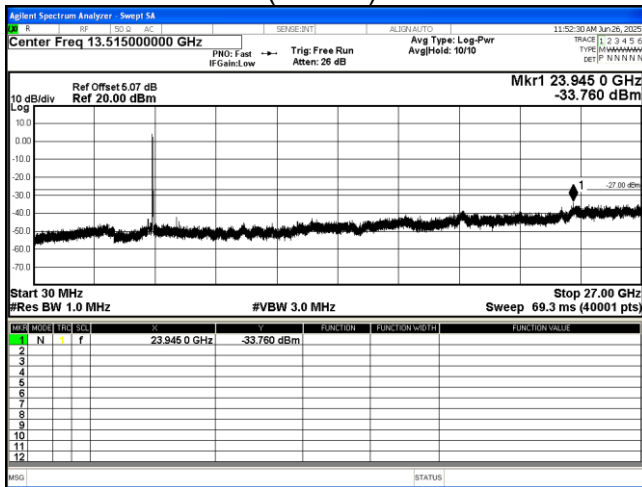
802.11 be(EHT40) 5310MHz
