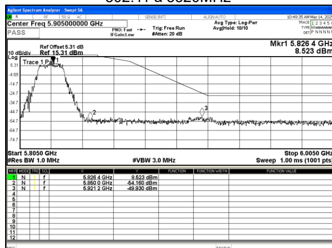
802.11 a 5825MHz
