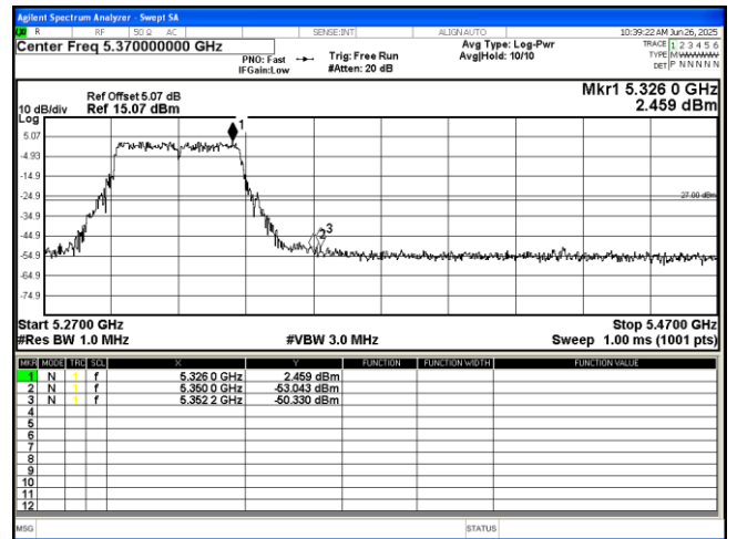
802.11 n40 5310MHz
