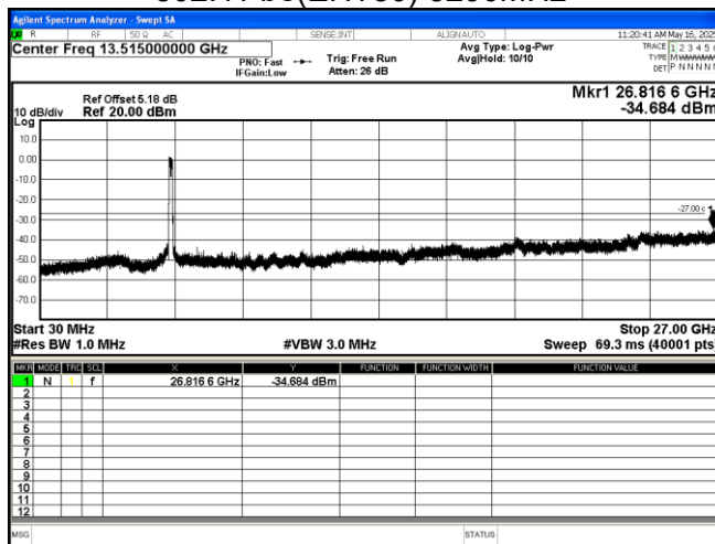
802.11 be(EHT160) 5250MHz
