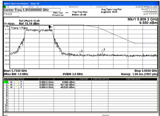
802.11 n40 5795MHz
