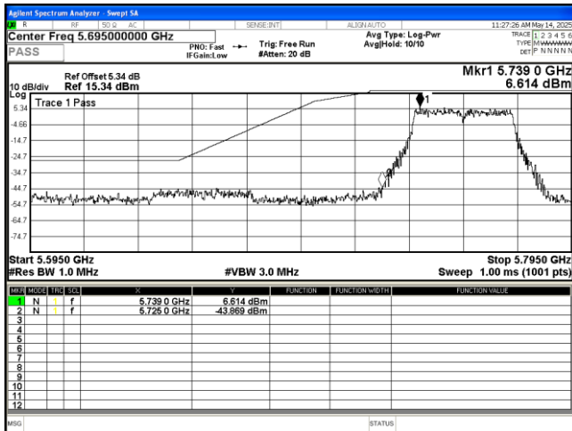
802.11 n40 5755MHz
