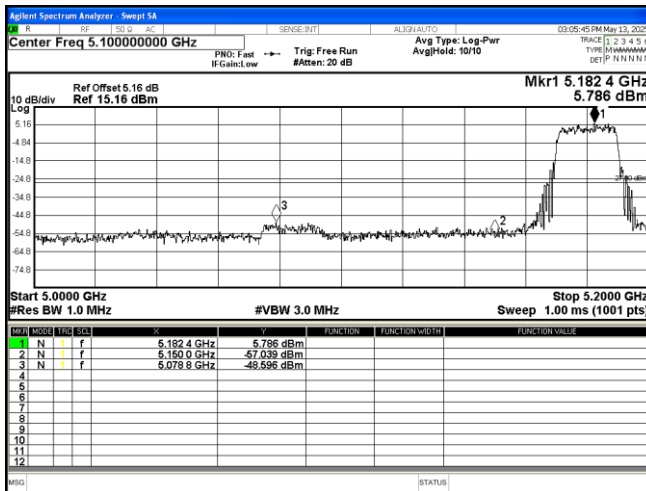
802.11 ax(HE20) 5180MHz
