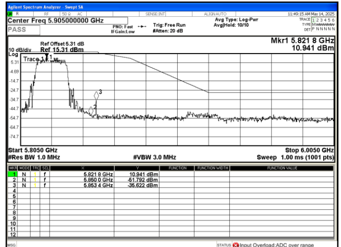
802.11 ax(HE20) 5825MHz
