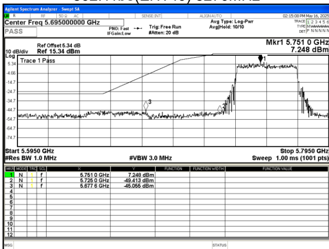
802.11 be(EHT40) 5755MHz
