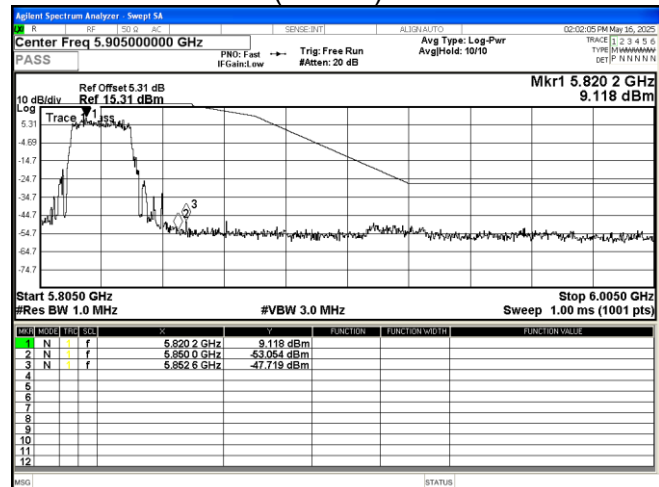
802.11be(EHT20) 5825MHz
