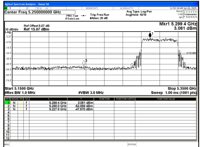
802.11 be(EHT40) 5310MHz
