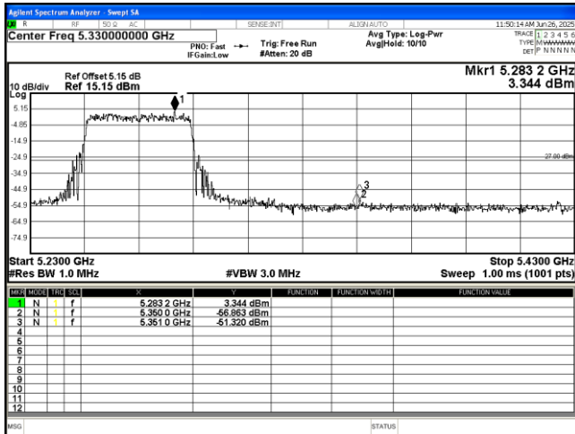
802.11be(EHT40) 5270MHz
