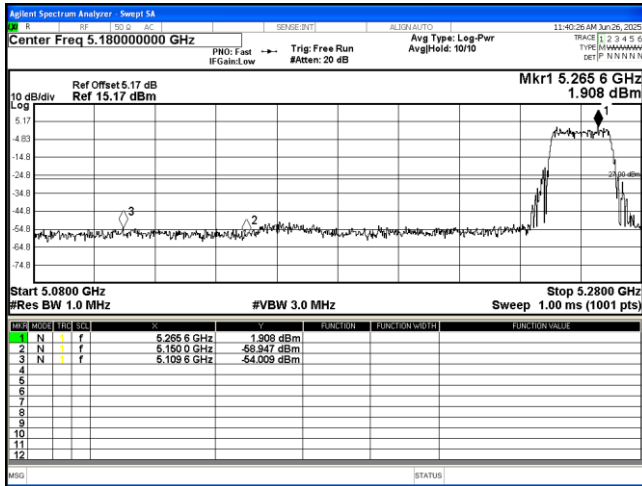
802.11 be(EHT20) 5260MHz
