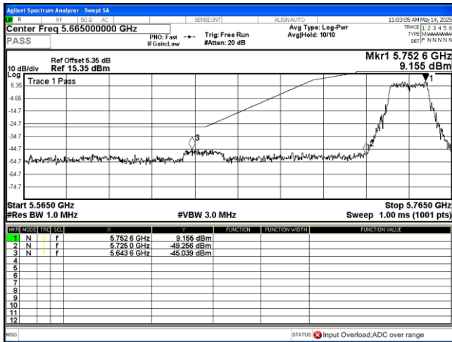
802.11 n20 5745MHz
