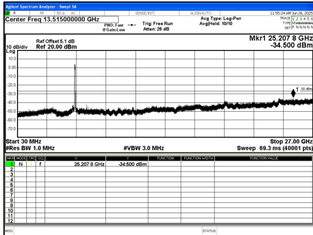
802.11 be(EHT80) 5290MHz
