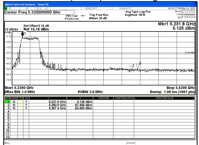
802.11 be(EHT20) 5240MHz
