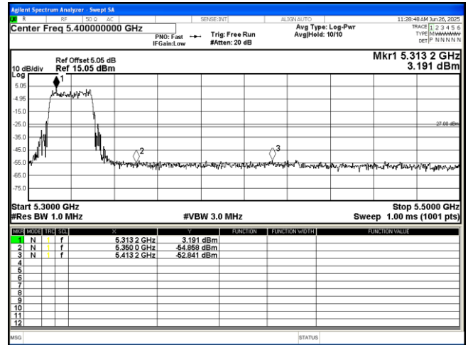
802.11 be(EHT20) 5320MHz
