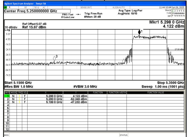
802.11 ax(HE40) 5310MHz
