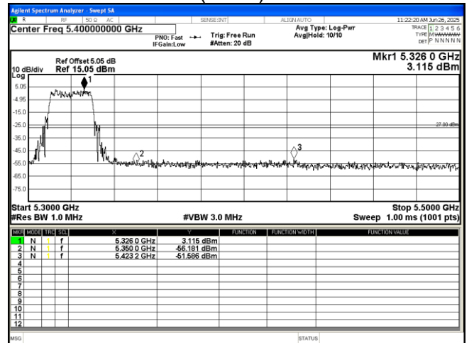
802.11 ax(HE20) 5320MHz
