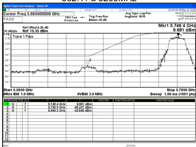
802.11 a 5745MHz
