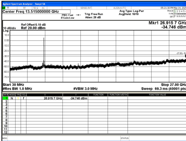
802.11 be(EHT40) 5230MHz
