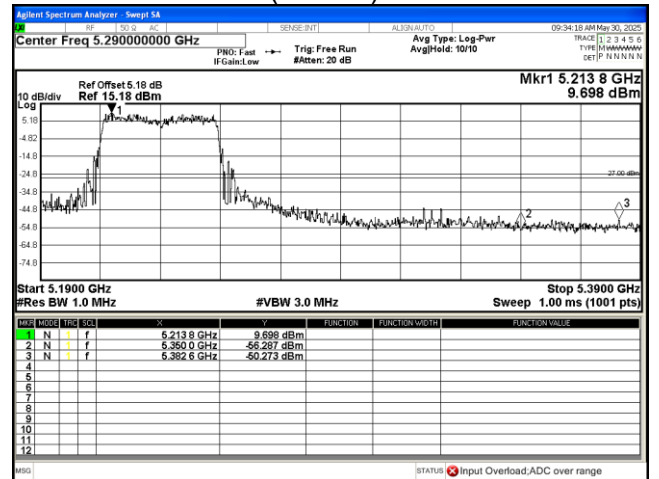
802.11 be(EHT40) 5230MHz
