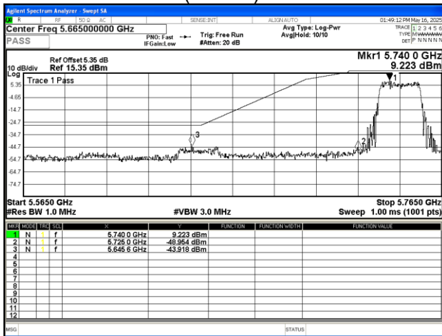
802.11 be(EHT20) 5745MHz
