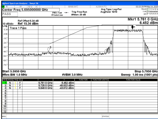
802.11 ax(HE40) 5755MHz
