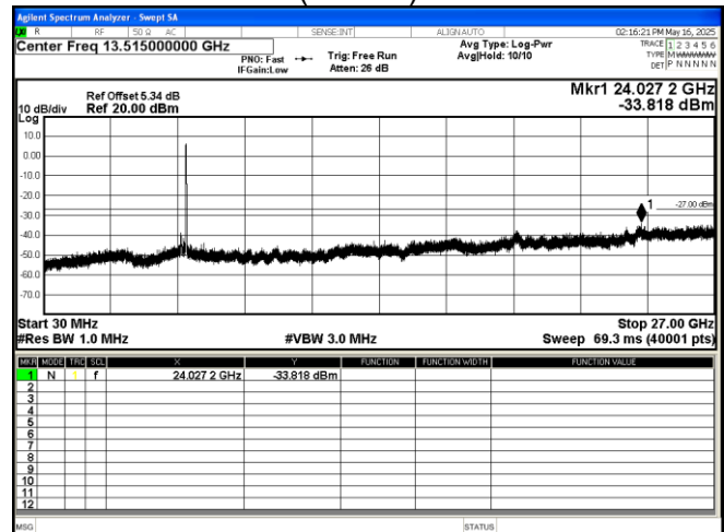
802.11 be(EHT40) 5270MHz
