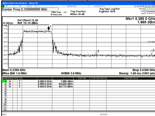
802.11 ax(HE40) 5270MHz
