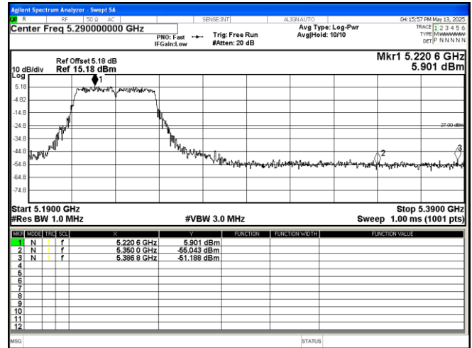
802.11 n40 5230MHz
