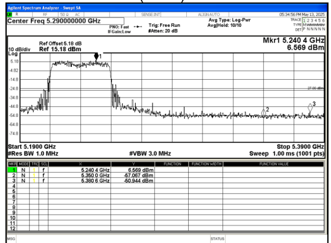
802.11 ax(HE40) 5230MHz
