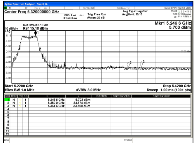
802.11 ac20 5240MHz
