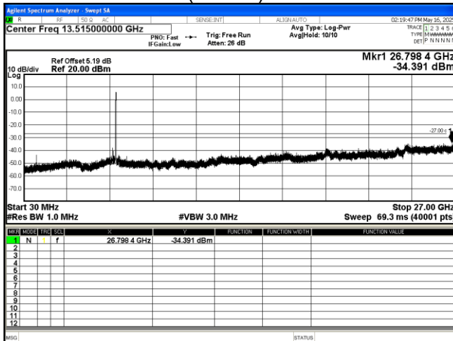
802.11 be(EHT40) 5310MHz
