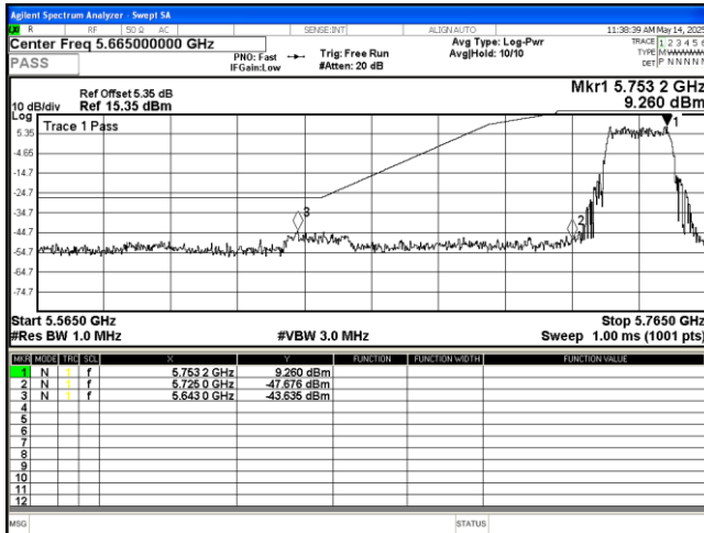
802.11 ax(HE20) 5745MHz
