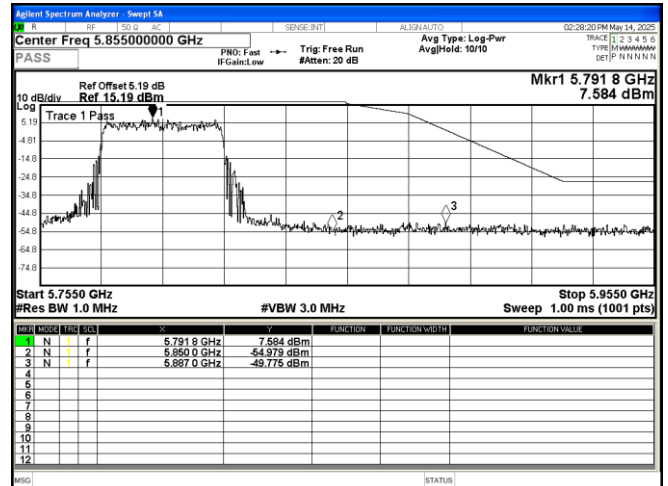
802.11 ax(HE40) 5795MHz
