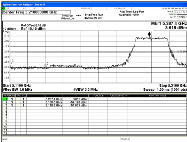
802.11 n40 5270MHz
