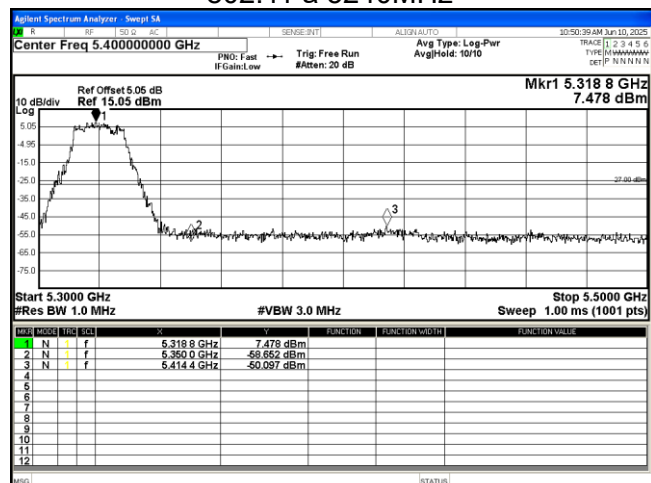
802.11 a 5320MHz
