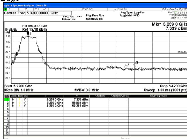
802.11 a 5240MHz
