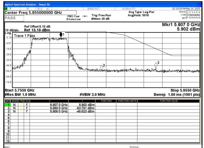
802.11 ac40 5795MHz
