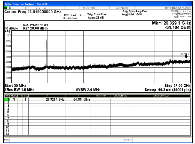
802.11 be(EHT40) 5270MHz
