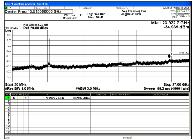
802.11 be(EHT80) 5775MHz
