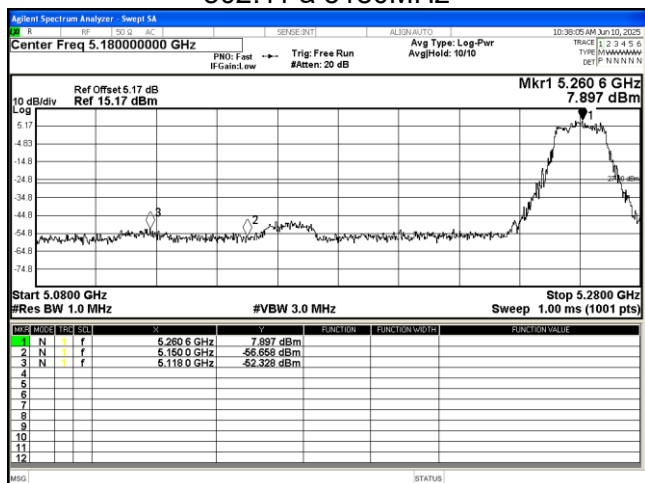
802.11 a 5260MHz
