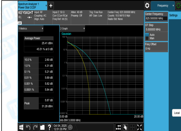
Band26(824-849)-3MHz-QPSK-26915-1RB#0-PASS
