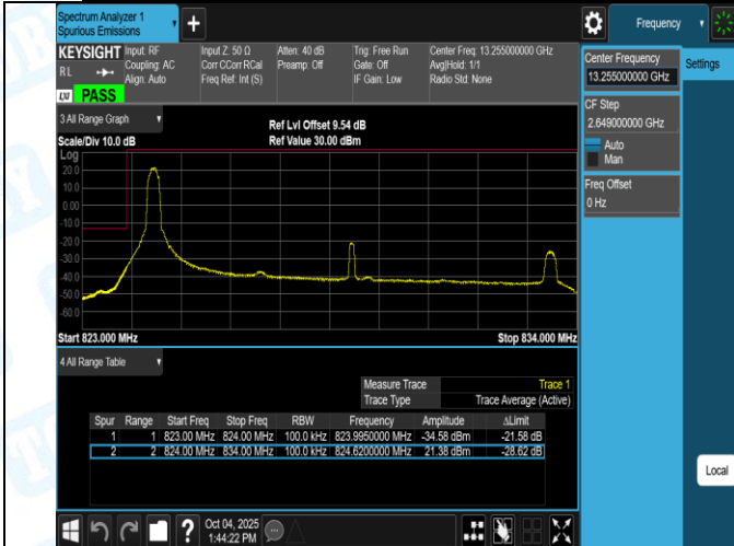
Band26(824-849)-10MHz-QPSK-26840-50RB#0-PASS
