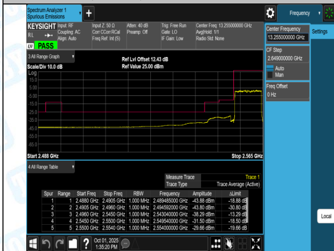
Band41(2555-2655)-10MHz-QPSK-41190-1RB#49-PASS
