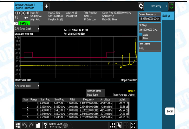
Band41(2555-2655)-10MHz-QPSK-41190-1RB#0-PASS
