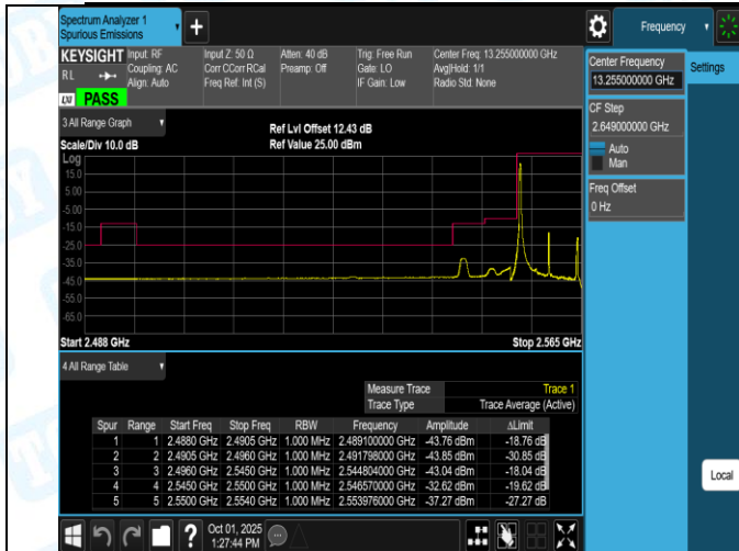
Band41(2555-2655)-10MHz-QPSK-40290-50RB#0-PASS
