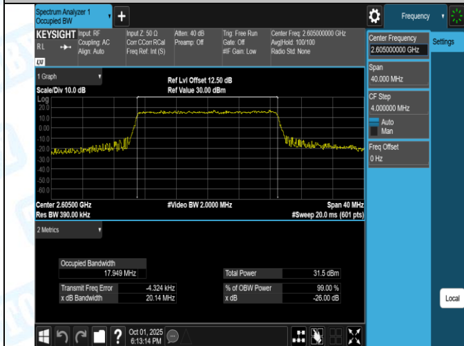
Band41(2555-2655)-20MHz-16QAM-40740-100RB#0-PASS
