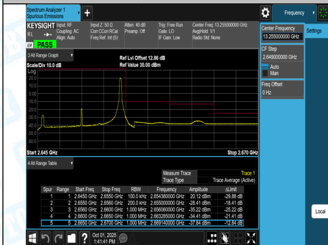
Band41(2555-2655)-10MHz-16QAM-40290-1RB#0-PASS
