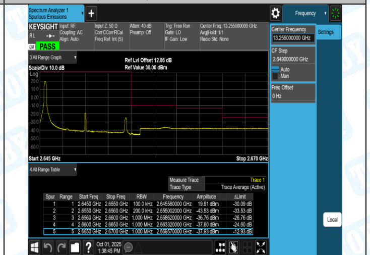
Band41(2555-2655)-10MHz-QPSK-41190-50RB#0-PASS
