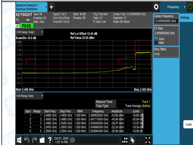
Band41(2555-2655)-10MHz-16QAM-41190-1RB#49-PASS
