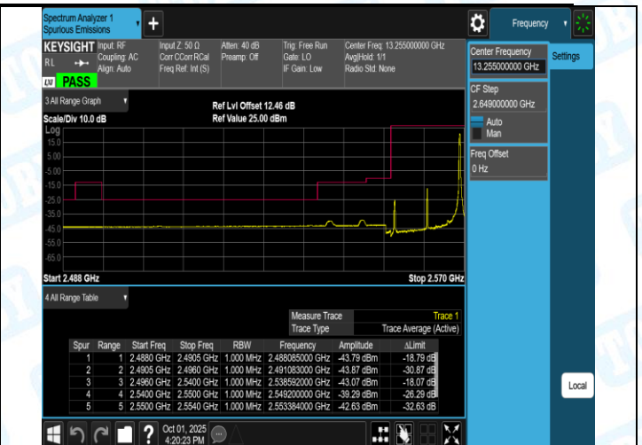
Band41(2555-2655)-15MHz-QPSK-41165-1RB#0-PASS
