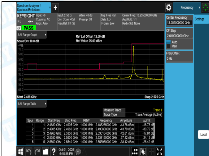
Band41(2555-2655)-20MHz-QPSK-40340-100RB#0-PASS
