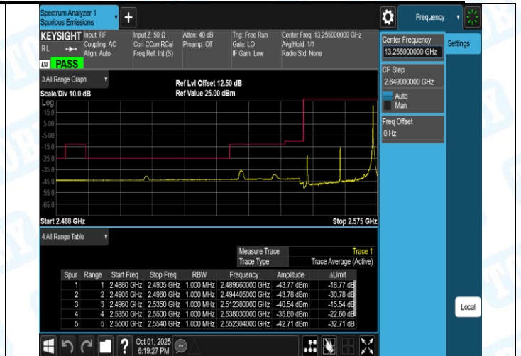
Band41(2555-2655)-20MHz-QPSK-41140-1RB#0-PASS
