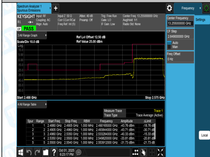
Band41(2555-2655)-20MHz-QPSK-41140-1RB#99-PASS
