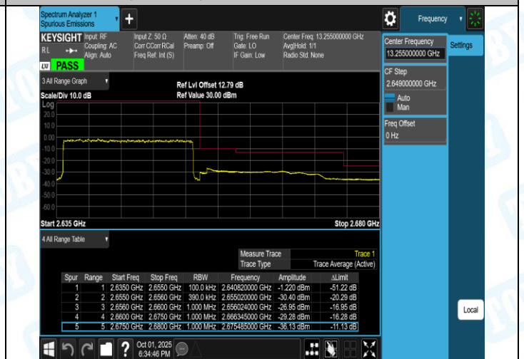
Band41(2555-2655)-20MHz-16QAM-40340-1RB#99-PASS
