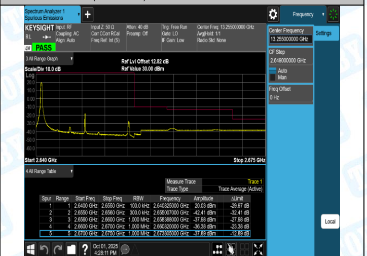
Band41(2555-2655)-15MHz-QPSK-41165-75RB#0-PASS
