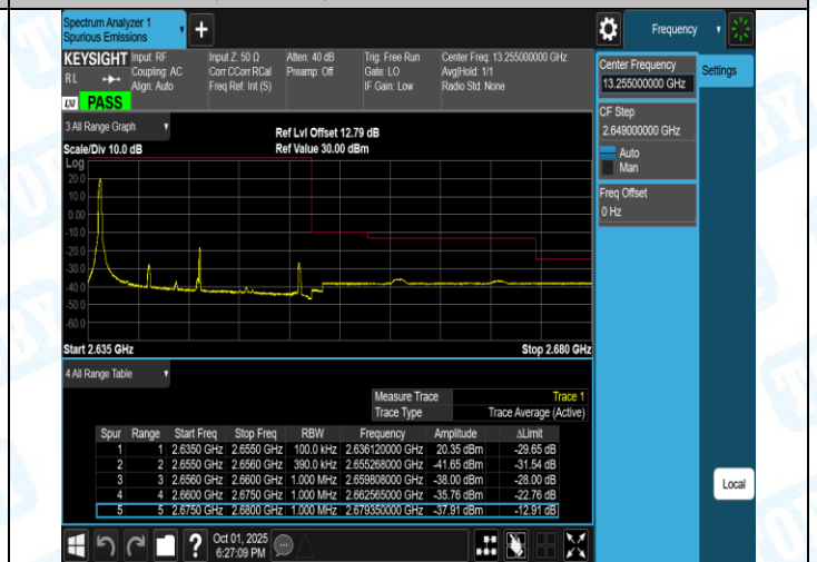
Band41(2555-2655)-20MHz-QPSK-41140-100RB#0-PASS
