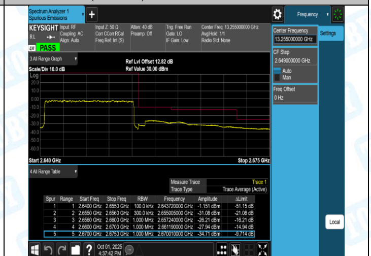
Band41(2555-2655)-20MHz-QPSK-40340-1RB#99-PASS
