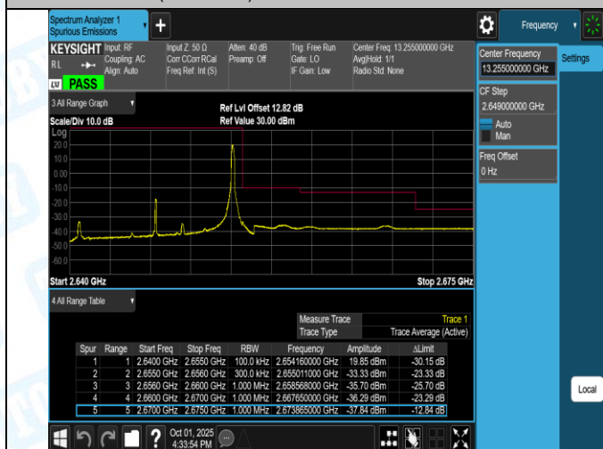
Band41(2555-2655)-20MHz-QPSK-40340-1RB#0-PASS
