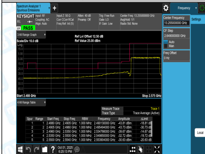
Band41(2555-2655)-20MHz-16QAM-41140-1RB#99-PASS
