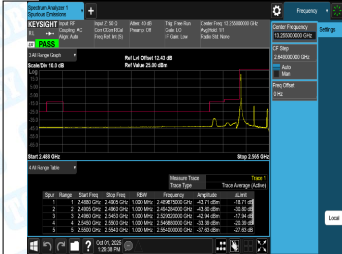
Band41(2555-2655)-10MHz-16QAM-40290-50RB#0-PASS
