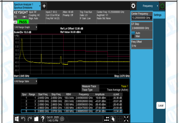
Band41(2555-2655)-10MHz-16QAM-41190-50RB#0-PASS
