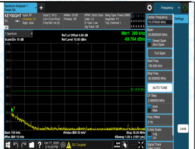
Band41(2555-2655)-10MHz-16QAM-40740-1RB#0-1000-3000-PASS
