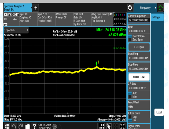
Band41(2555-2655)-10MHz-16QAM-40740-50RB#0-0.15~30-PASS
