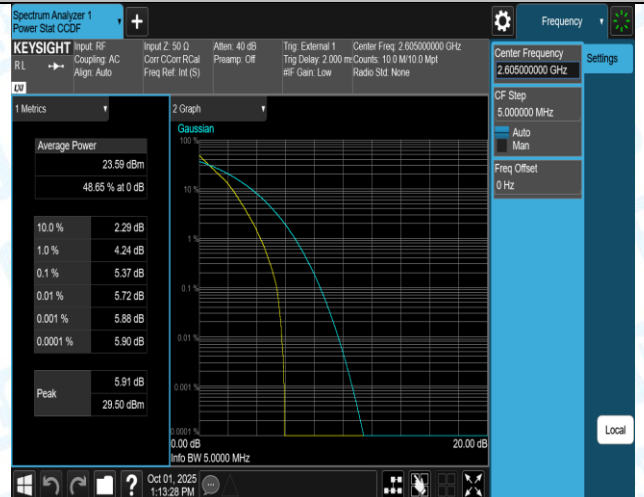
Band41(2555-2655)-5MHz-QPSK-41215-25RB#0-PASS
