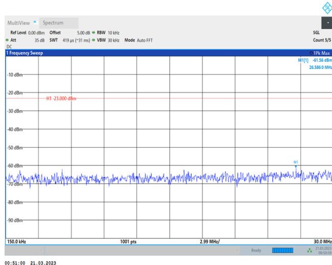
Band43-20MHz-QPSK-44690-1RB#0-Range2:0.15~30MHz
