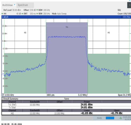
Band48-10MHz-QPSK-55290-50RB#0-PASS
