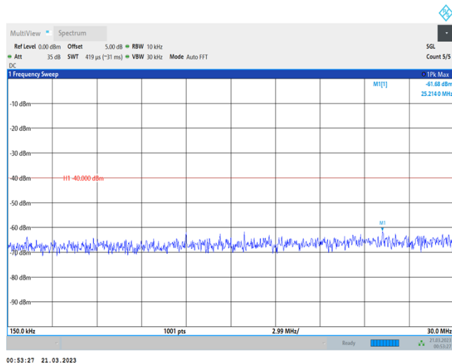
Band48-20MHz-QPSK-55340-1RB#0-Range2:0.15~30MHz
