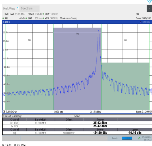
Band48-10MHz-QPSK-56690-1RB#49-PASS
