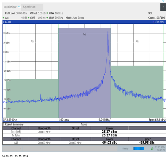
Band48-20MHz-QPSK-56640-1RB#99-PASS
