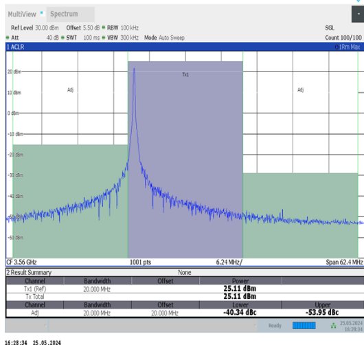
Band48-20MHz-QPSK-55340-1RB#0-PASS
