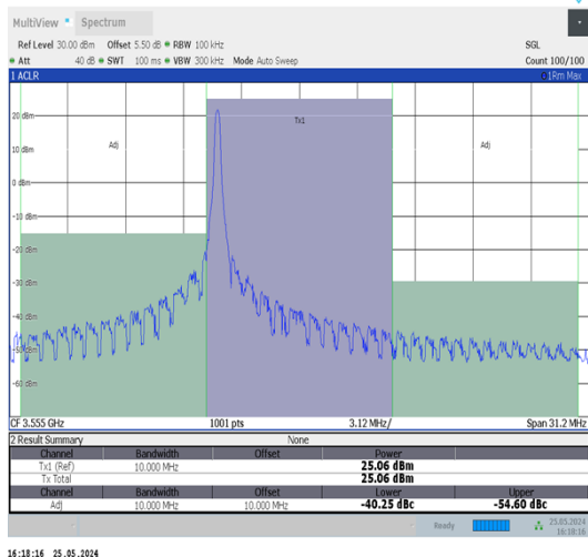
Band48-10MHz-QPSK-55290-1RB#0-PASS
