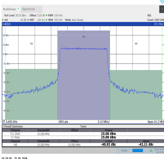
Band48-10MHz-QPSK-56690-50RB#0-PASS
