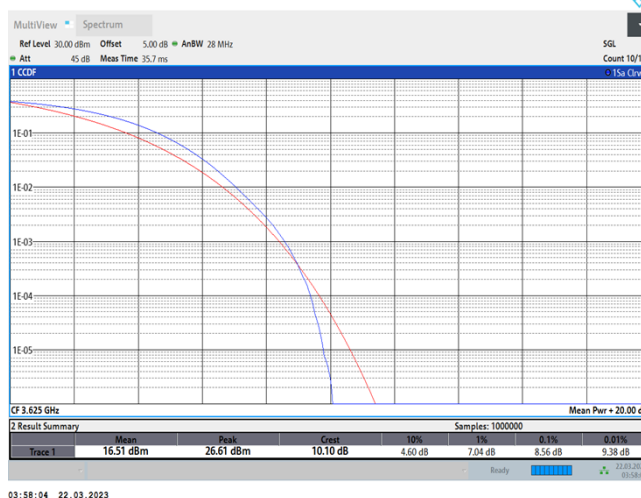
48-48-20MHz-20MHz-QPSK-QPSK-55891-56089-100RB#0-100RB#0
