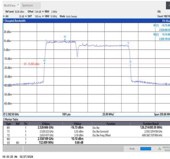
NTVN_CA_n41C_PC3_30+30_50+80_M+M_Ant1_TID1_1_#1
