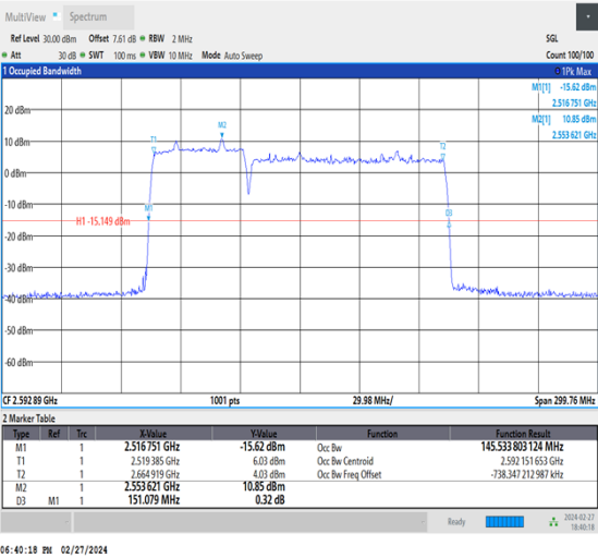
NTNV_CA_n41C_PC3_30+30_50+100_M+M_Ant1_TID3 _1_#1
