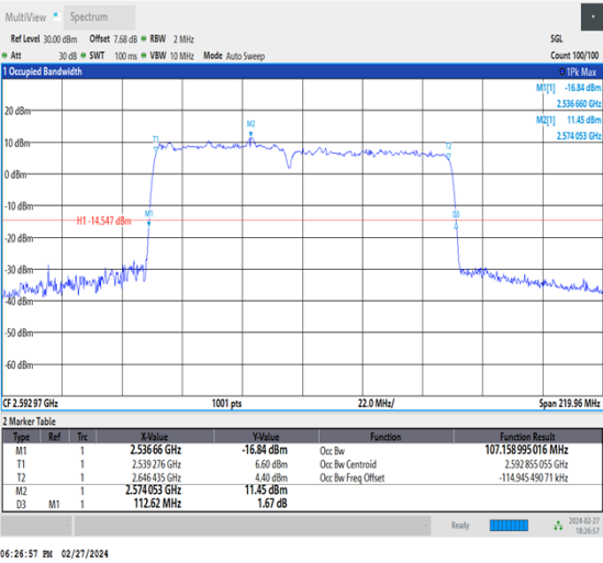
NTVN_CA_n41C_PC3_30+30_50+60_M+M_Ant1_TID7_1_#1
