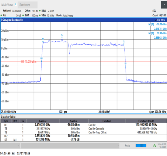
NTNV_CA_n41C_PC3_30+30_50+100_M+M_Ant1_TID1 _1_#1
