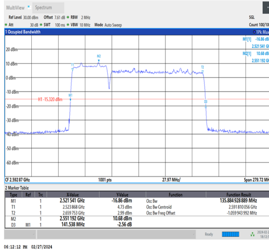
NTNV_CA_n41C_PC3_30+30_40+100_M+M_Ant1_TID9_1_#1
