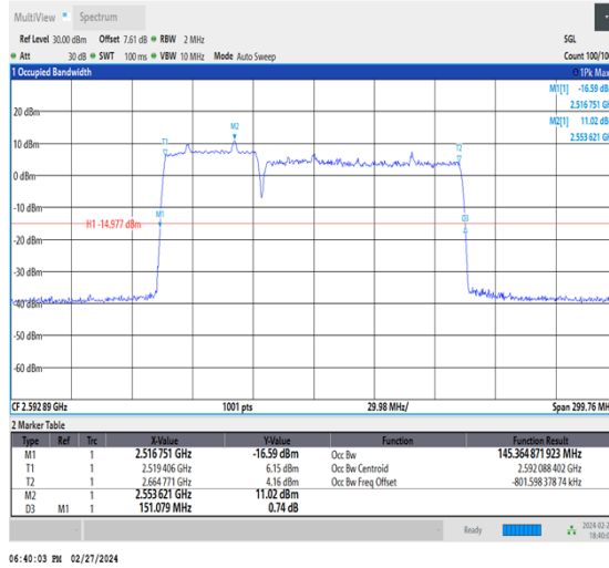
NTNV_CA_n41C_PC3_30+30_50+100_M+M_Ant1_TID2 _1_#1
