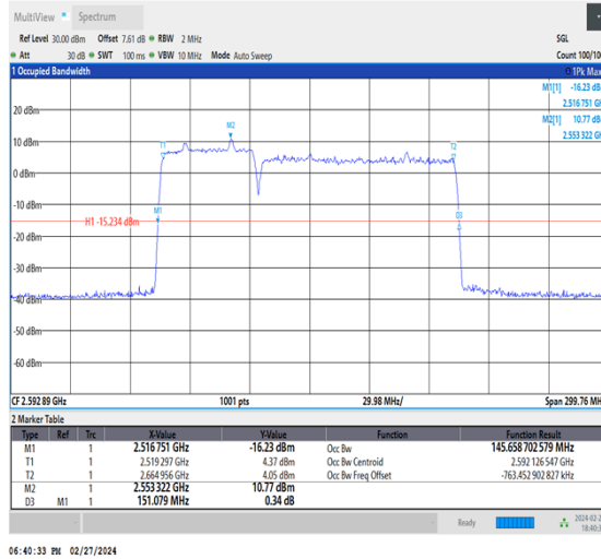
NTNV_CA_n41C_PC3_30+30_50+100_M+M_Ant1_TID4 _1_#1
