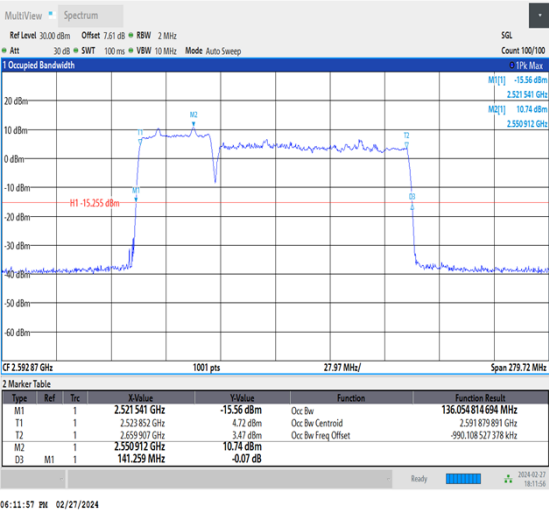
NTNV_CA_n41C_PC3_30+30_40+100_M+M_Ant1_TID8_1_#1
