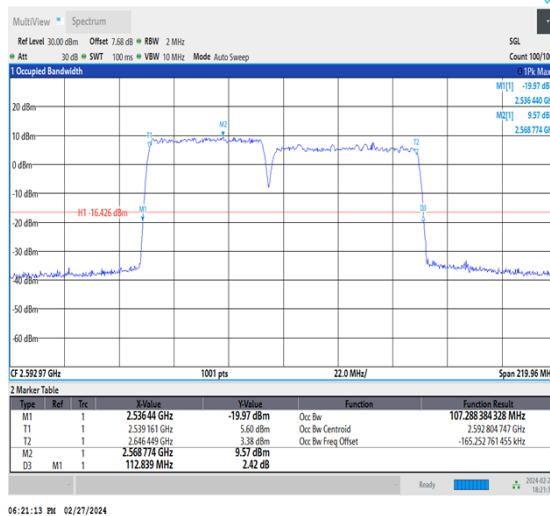
NTNV_CA_n41C_PC3_30+30_50+60_M+M_Ant1_TID2_1_#1
