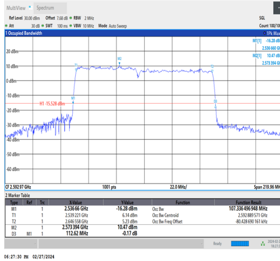
NTVN_CA_n41C_PC3_30+30_50+60_M+M_Ant1_TID8_1_#1
