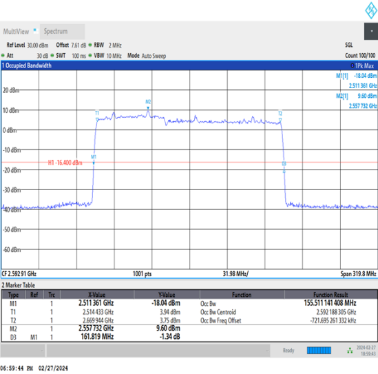
NTNV_CA_n41C_PC3_30+30_60+100_M+M_Ant1_TID2 _1_#1
