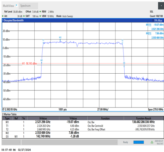
NTNV_CA_n41C_PC3_30+30_60+80_M+M_Ant1_TID9_1_#1
