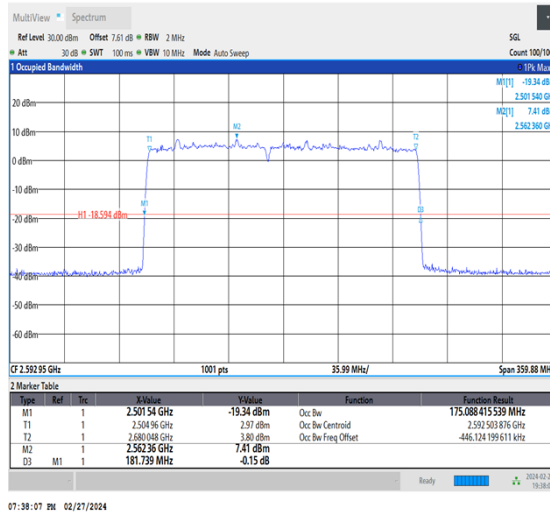
NTNV_CA_n41C_PC3_30+30_80+100_M+M_Ant1_TID3_1_#1
