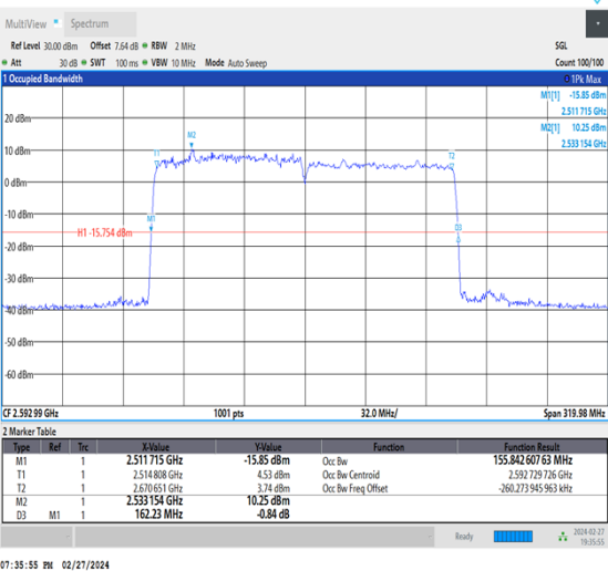
NTNV_CA_n41C_PC3_30+30_80+80_M+M_Ant1_TID9_1_#1
