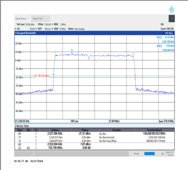
NTVN_CA_n41C_PC3_30+30_60+80_M+M_Ant1_TID3_1_#1
