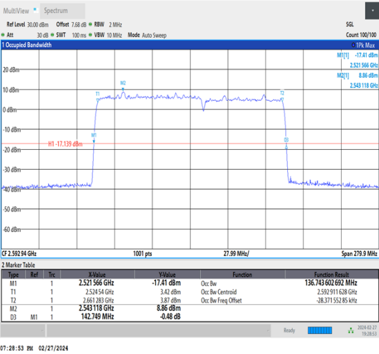
NTNV_CA_n41C_PC3_30+30_80+60_M+M_Ant1_TID9_1_#1
