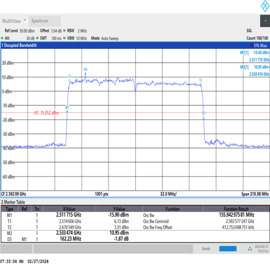
NTNV_CA_n41C_PC3_30+30_80+80_M+M_Ant1_TID1_1_#1
