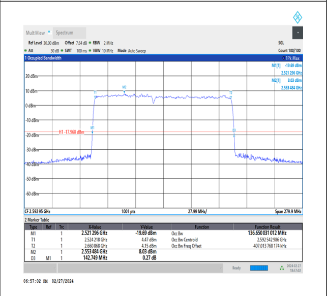
NTVN_CA_n41C_PC3_30+30_60+80_M+M_Ant1_TID6_1_#1
