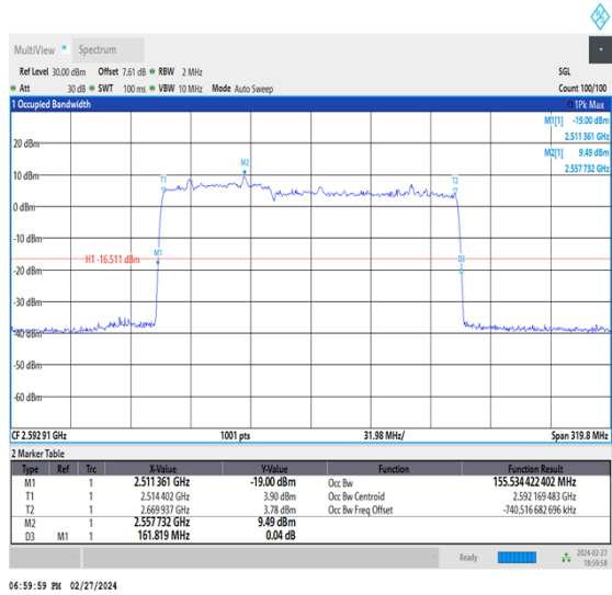
NTNV_CA_n41C_PC3_30+30_60+100_M+M_Ant1_TID3 _1_#1
