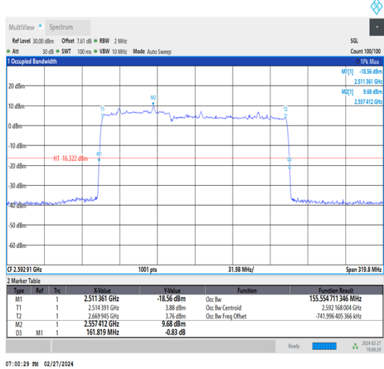
NTNV_CA_n41C_PC3_30+30_60+100_M+M_Ant1_TID5 _1_#1
