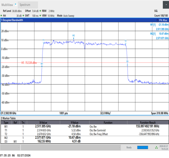
NTNV_CA_n41C_PC3_30+30_80+80_M+M_Ant1_TID7_1_#1
