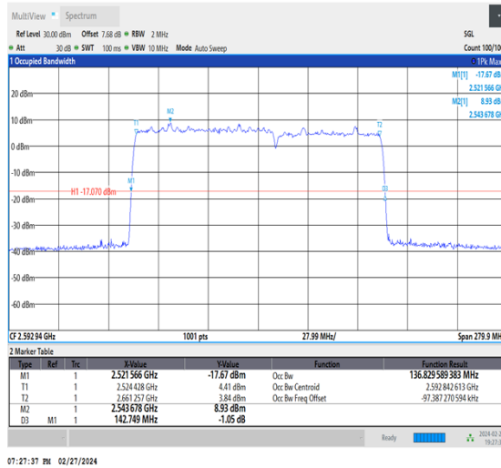
NTNV_CA_n41C_PC3_30+30_80+60_M+M_Ant1_TID4_1_#1
