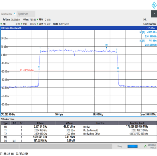
NTNV_CA_n41C_PC3_30+30_80+100_M+M_Ant1_TID8_1_#1
