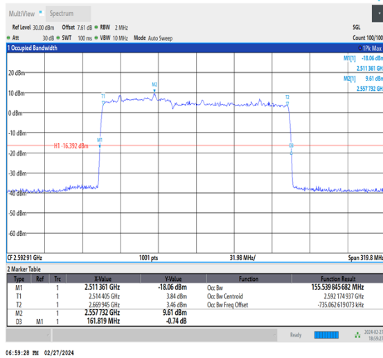
NTNV_CA_n41C_PC3_30+30_60+100_M+M_Ant1_TID1_1_#1
