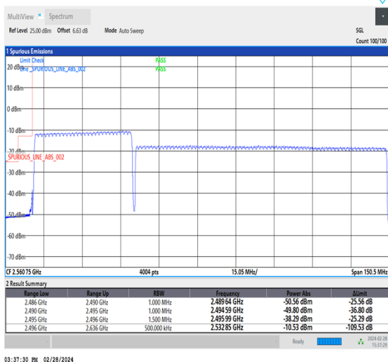
NTNV_CA_n41C_PC3_30+30_40+100_L+L_TID6_1_#1
