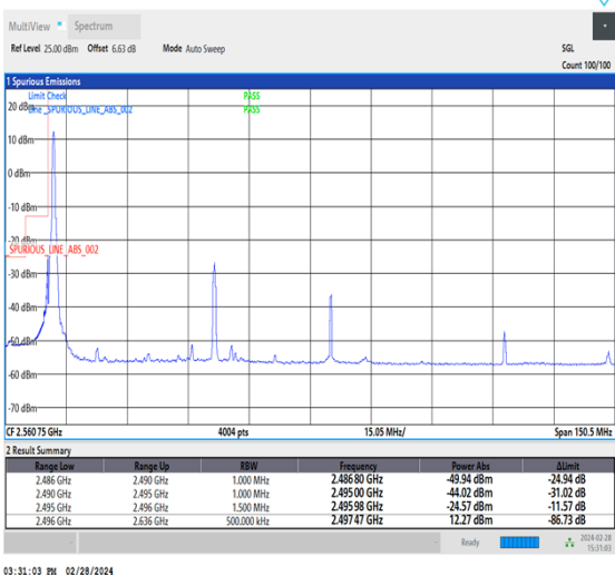
NTNV_CA_n41C_PC3_30+30_40+100_L+L_TID4_1_#1
