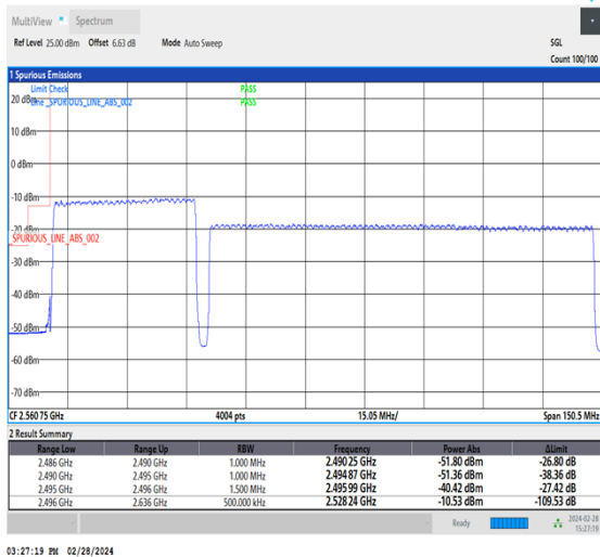
NTNV_CA_n41C_PC3_30+30_40+100_L+L_TID3_1_#1
