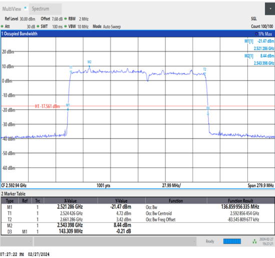
NTNV_CA_n41C_PC3_30+30_80+60_M+M_Ant1_TID3_1_#1
