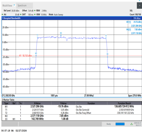
NTNV_CA_n41C_PC3_30+30_60+80_M+M_Ant1_TID7_1_#1
