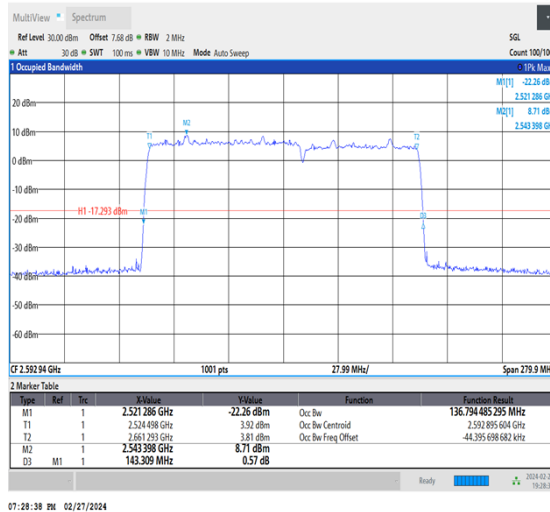
NTNV_CA_n41C_PC3_30+30_80+60_M+M_Ant1_TID8_1_#1
