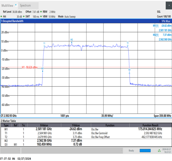
NTNV_CA_n41C_PC3_30+30_80+100_M+M_Ant1_TID2_1_#1
