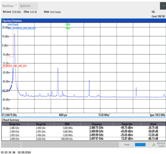
NTNV_CA_n41C_PC3_30+30_40+100_L+L_TID1_1_#1
