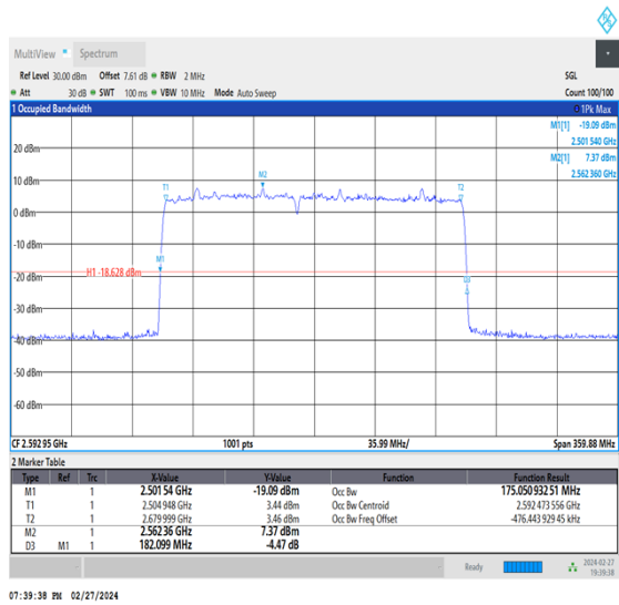
NTNV_CA_n41C_PC3_30+30_80+100_M+M_Ant1_TID9_1_#1
