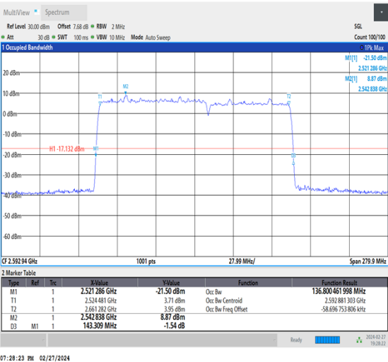
NTNV_CA_n41C_PC3_30+30_80+60_M+M_Ant1_TID7_1_#1
