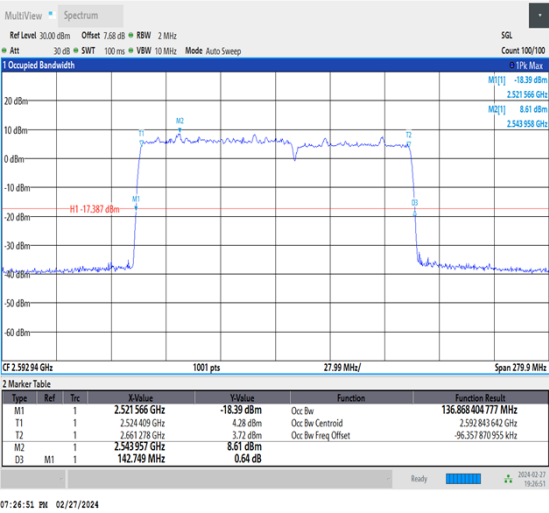
NTNV_CA_n41C_PC3_30+30_80+60_M+M_Ant1_TID1_1_#1
