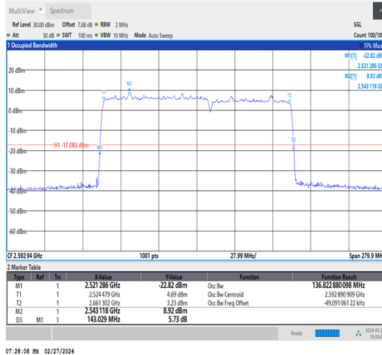
NTNV_CA_n41C_PC3_30+30_80+60_M+M_Ant1_TID6_1_#1
