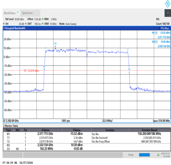
NTNV_CA_n41C_PC3_30+30_80+80_M+M_Ant1_TID2_1_#1
