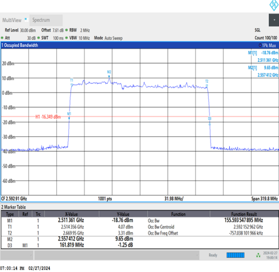
NTNV_CA_n41C_PC3_30+30_60+100_M+M_Ant1_TID4 _1_#1
