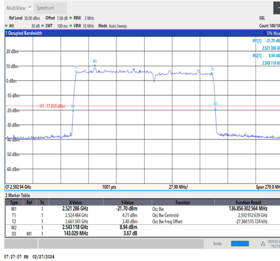
NTNV_CA_n41C_PC3_30+30_80+60_M+M_Ant1_TID2_1_#1
