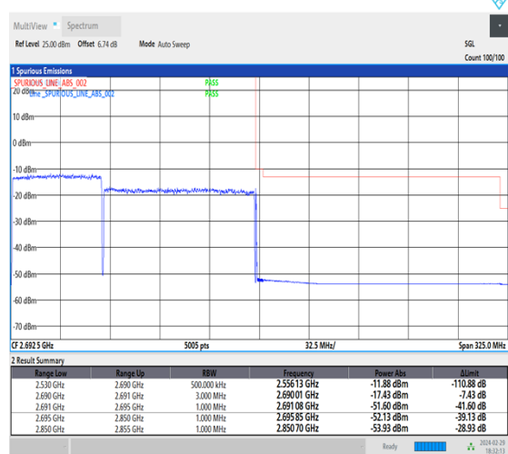
NTNV_CA_n41C_PC3_30+30_60+100_H+H_TID6_1_#1
