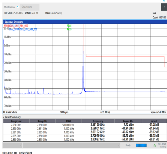
NTNV_CA_n41C_PC3_30+30_60+100_H+H_TID2_1_#1
