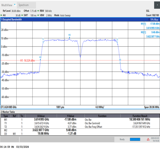
NTNV_CA_n48B_PC3_30+30_10+10_M+M_Ant0_TID7_1_#1
