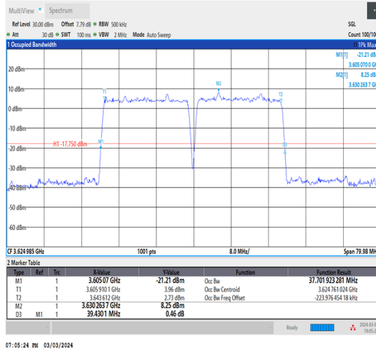
NTNV_CA_n48B_PC3_30+30_20+20_M+M_Ant0_TID2_1_#1
