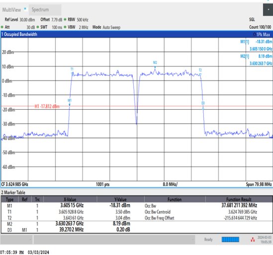
NTNV_CA_n48B_PC3_30+30_20+20_M+M_Ant0_TID3_1_#1
