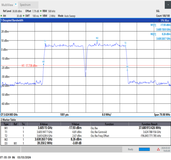
NTNV_CA_n48B_PC3_30+30_20+20_M+M_Ant0_TID1_1_#1
