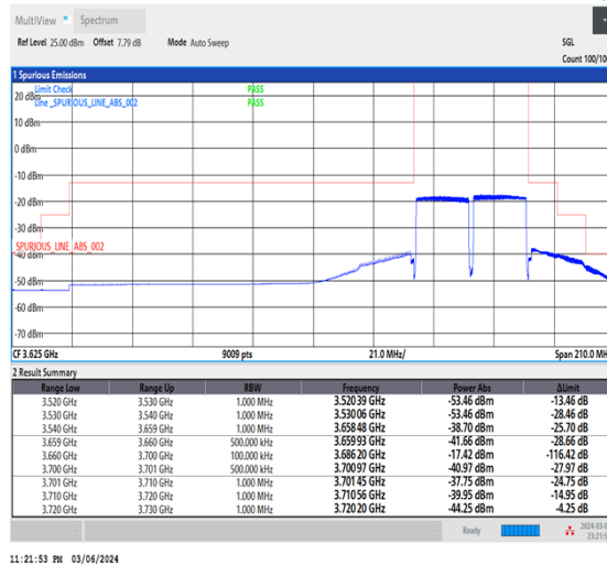
NTNV_CA_n48B_PC3_30+30_20+20_H+H_TID6_1_#1
