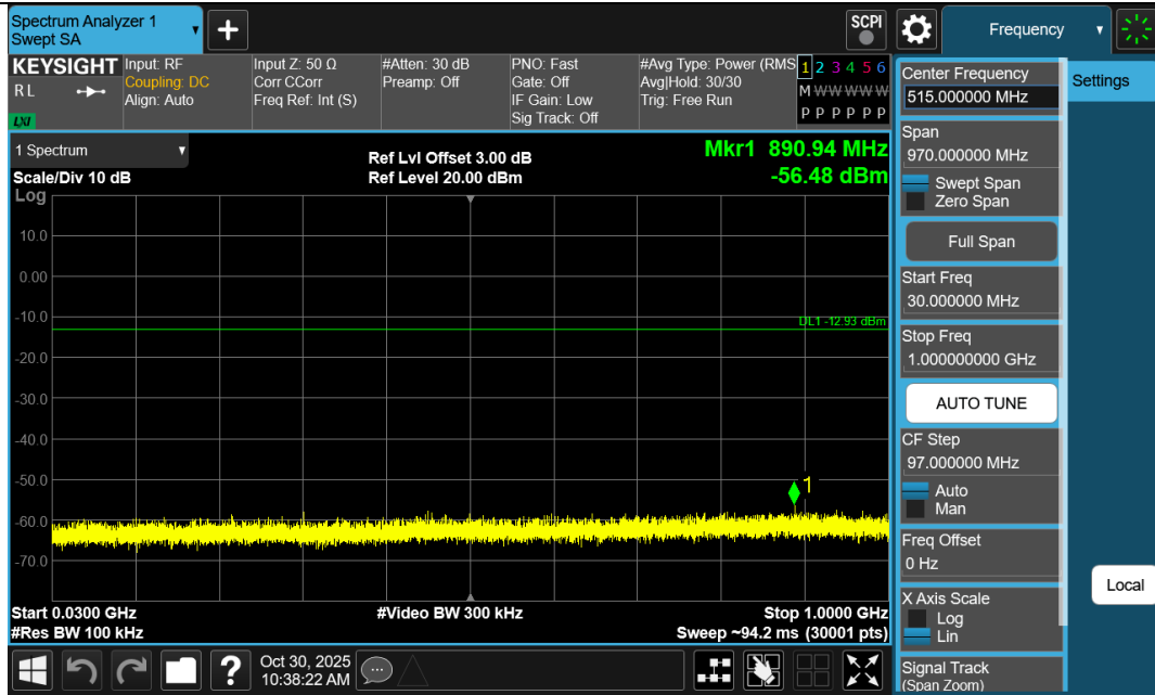
11G-Ant1-2412-30~1000-PASS
