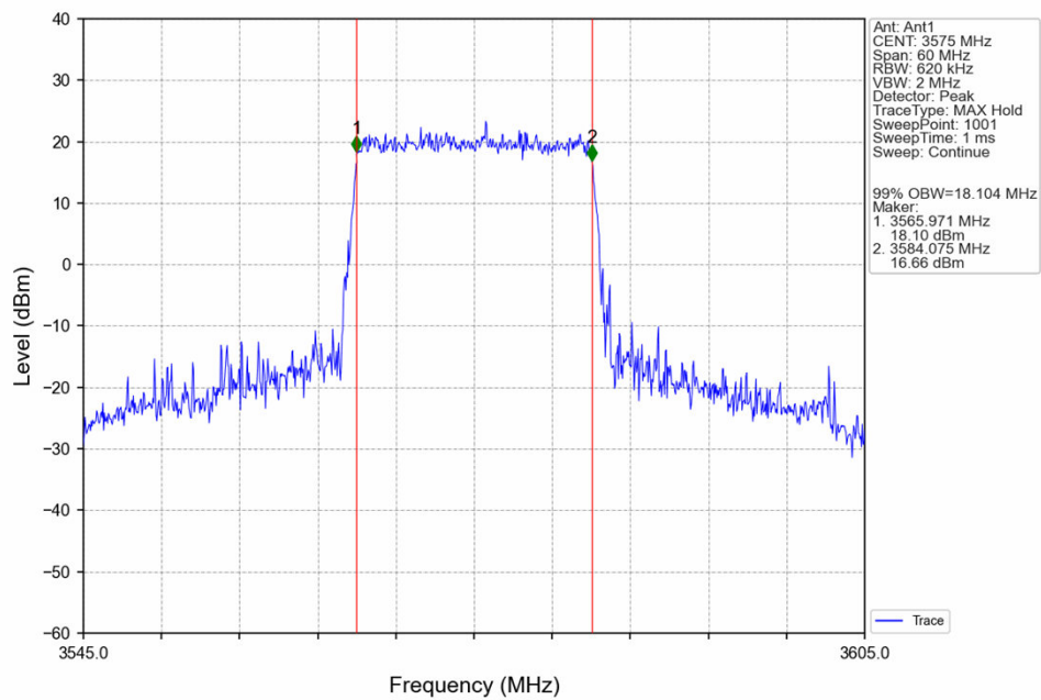
Band42c_20MHz_QPSK_MCH_3575MHz_RB_100_0_NTNV
