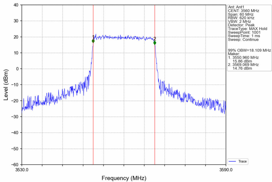
Band42c_20MHz_16QAM_LCH_3560MHz_RB_100_0_NTNV
