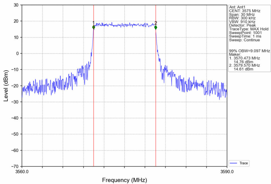
Band42c_10MHz_QPSK_MCH_3575MHz_RB_50_0_NTNV
