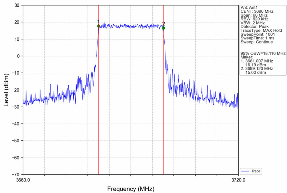
Band43c_20MHz_16QAM_HCH_3690MHz_RB_100_0_NTNV
