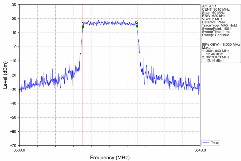
Band43c_20MHz_16QAM_LCH_3610MHz_RB_100_0_NTNV
