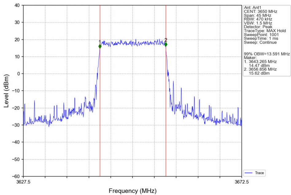
Band43c_15MHz_QPSK_MCH_3650MHz_RB_75_0_NTNV
