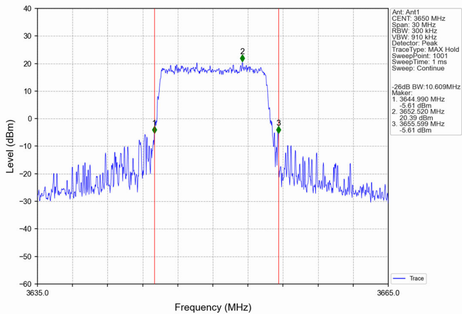
Band43c_10MHz_QPSK_MCH_3650MHz_RB_50_0_NTNV
