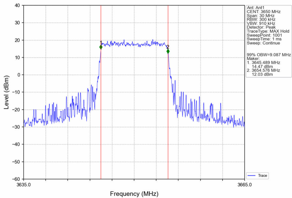
Band43c_10MHz_QPSK_MCH_3650MHz_RB_50_0_NTNV
