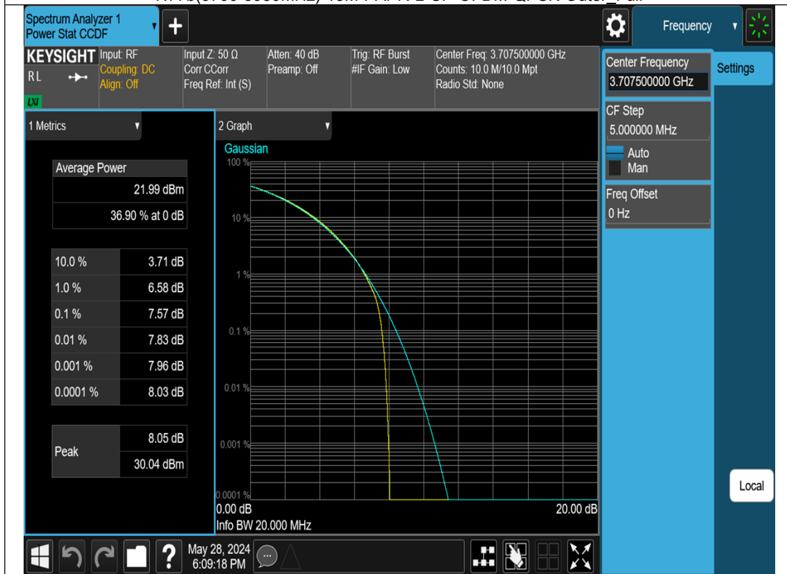
N77b(3700-3980MHz)-15M-PAPR-M-DFT-s-OFDM-Pi2 BPSK-Outer_Full
