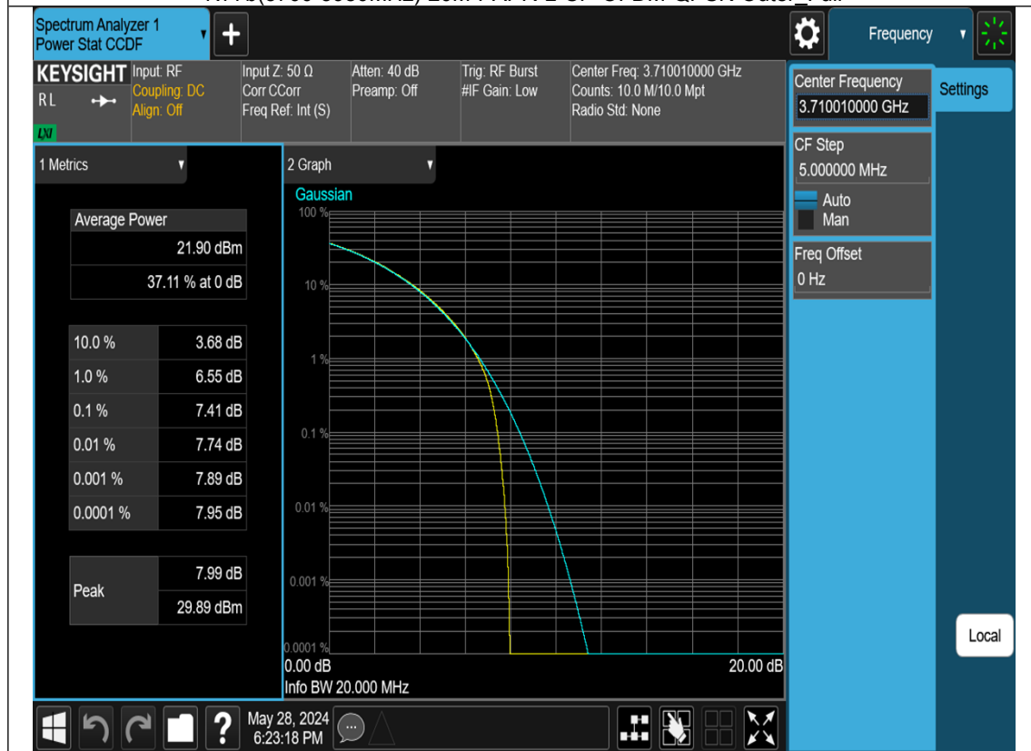
N77b(3700-3980MHz)-20M-PAPR-M-DFT-s-OFDM-Pi2 BPSK-Outer_Full
