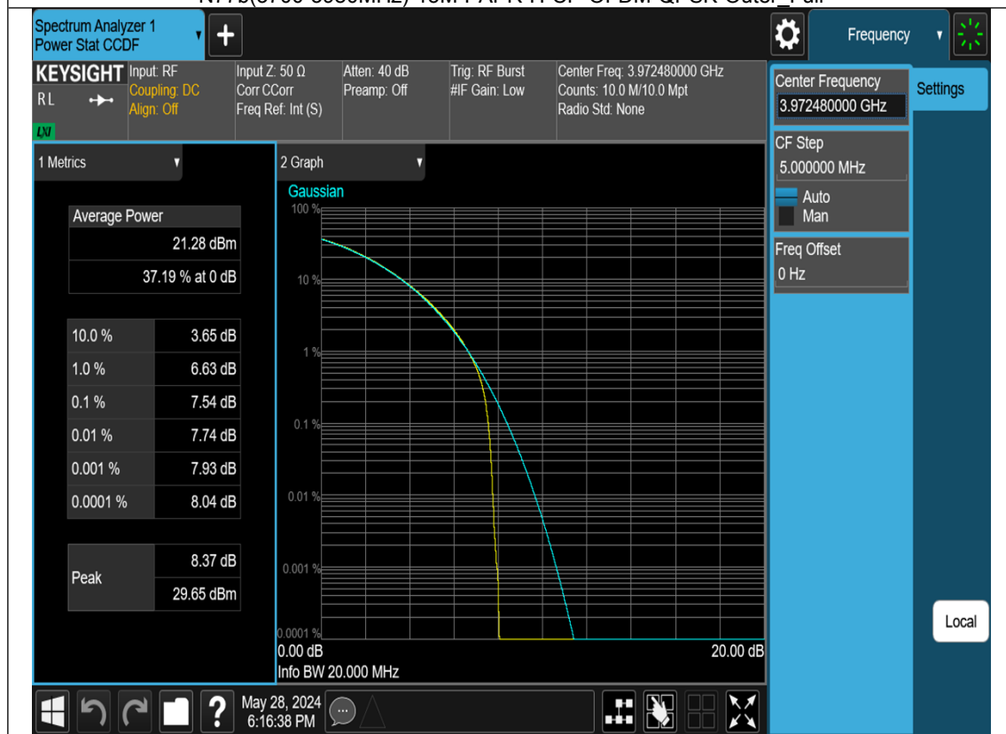
N77b(3700-3980MHz)-20M-PAPR-L-DFT-s-OFDM-Pi2 BPSK-Outer_Full
