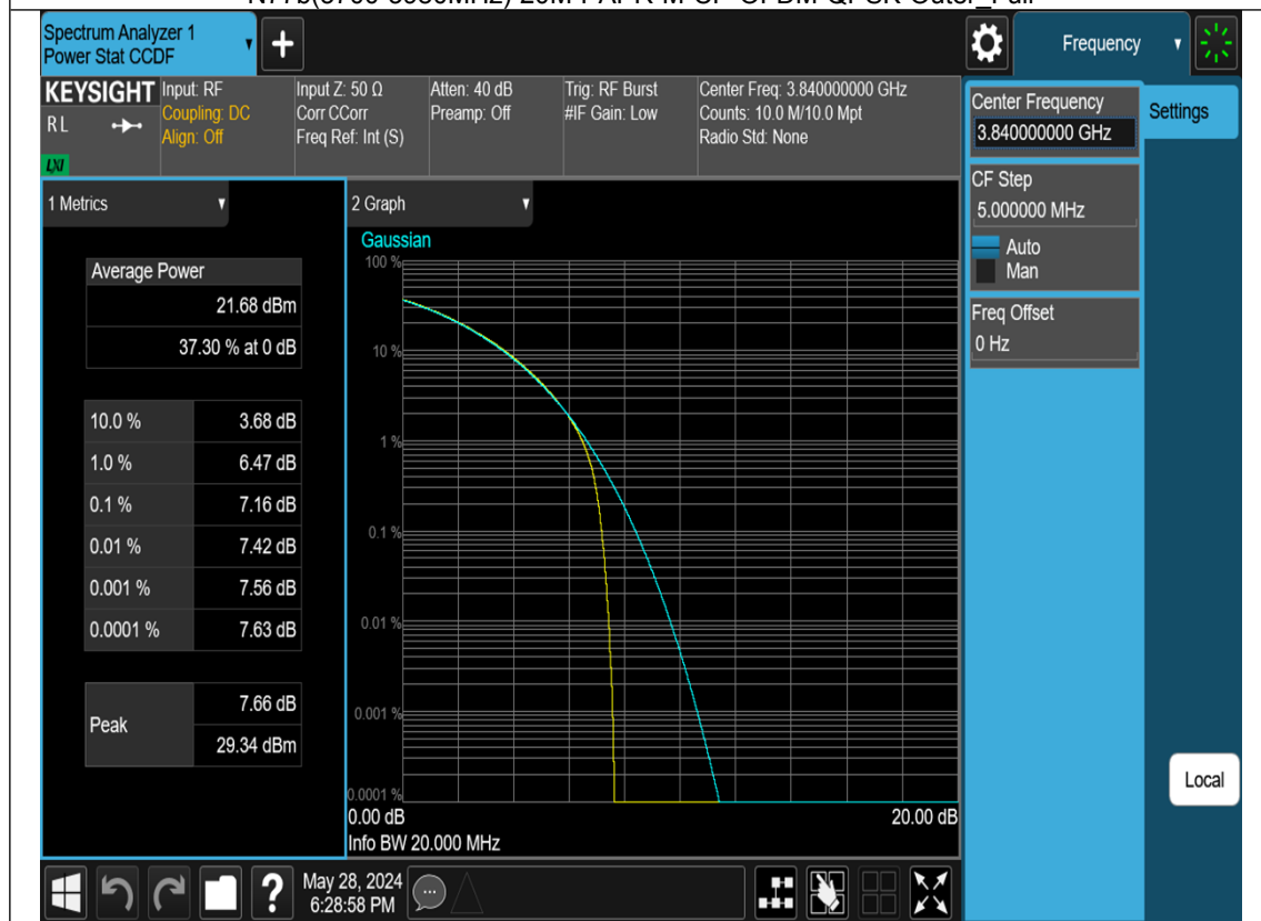
N77b(3700-3980MHz)-20M-PAPR-H-DFT-s-OFDM-Pi2 BPSK-Outer_Full
