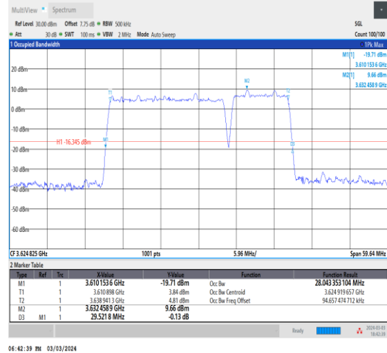
NTNV_CA_n48B_PC3_30+30_20+10_M+M_Ant0_TID4_1_#1
