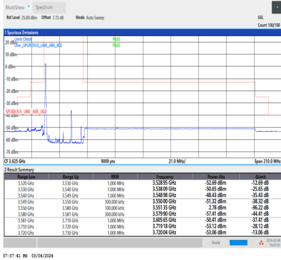
NTNV_CA_n48B_PC3_30+30_20+10_L+L_TID1_1_#1
