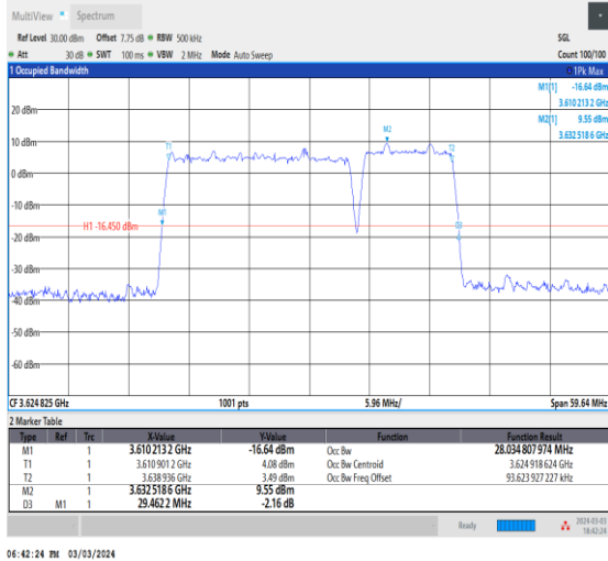
NTNV_CA_n48B_PC3_30+30_20+10_M+M_Ant0_TID3_1_#1
