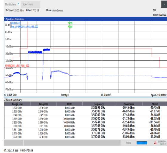
NTNV_CA_n48B_PC3_30+30_20+10_L+L_TID3_1_#1
