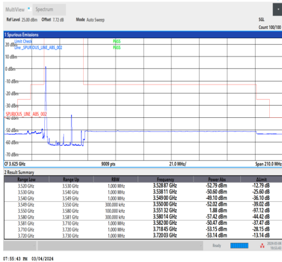
NTNV_CA_n48B_PC3_30+30_20+10_L+L_TID4_1_#1
