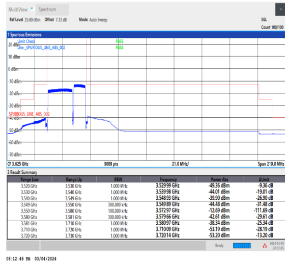
NTNV_CA_n48B_PC3_30+30_20+10_L+L_TID6_1_#1
