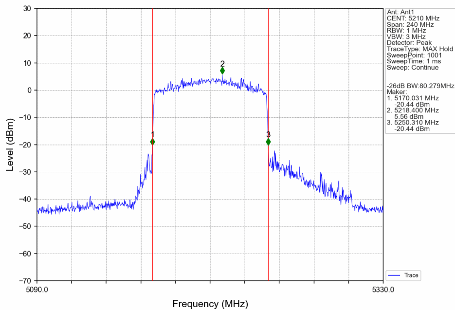
802.11be(EHT80)_MCH_5210MHz_SU_ / _Ant1_NTNV
