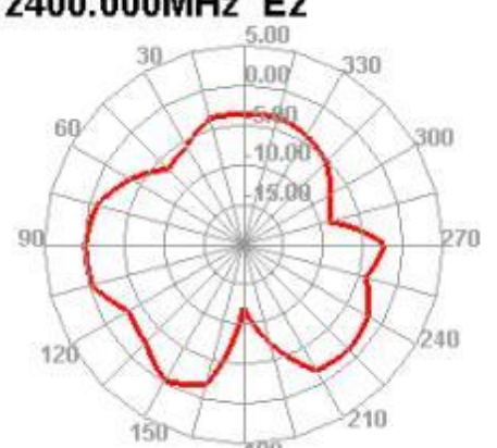
2400.000MHz E2
