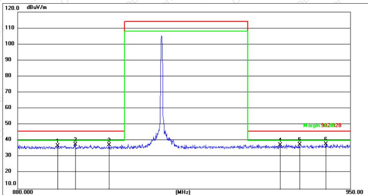
910.3MHz Horizontal
