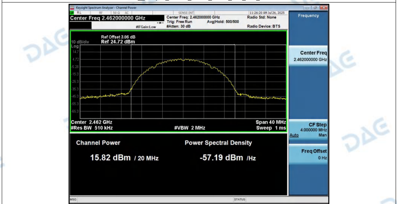
MAX__Output_Power_NVNT_ANT1_802_11b_2462
