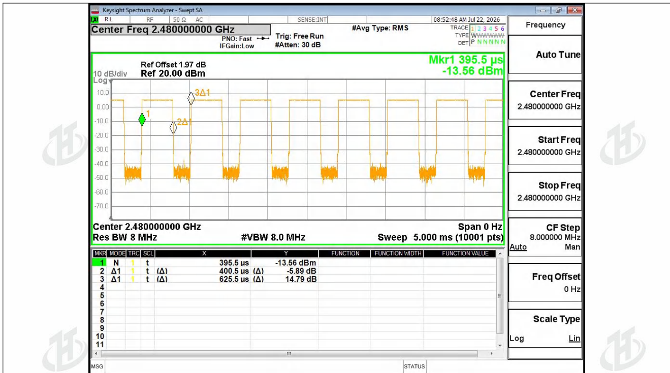
Duty Cycle NVNT BLE 1M 2480MHz Ant1
