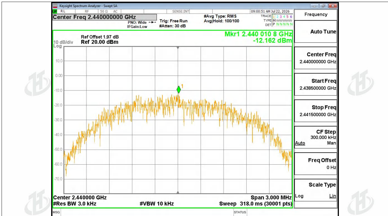
PSD NVNT BLE 2M 2440MHz Ant1
