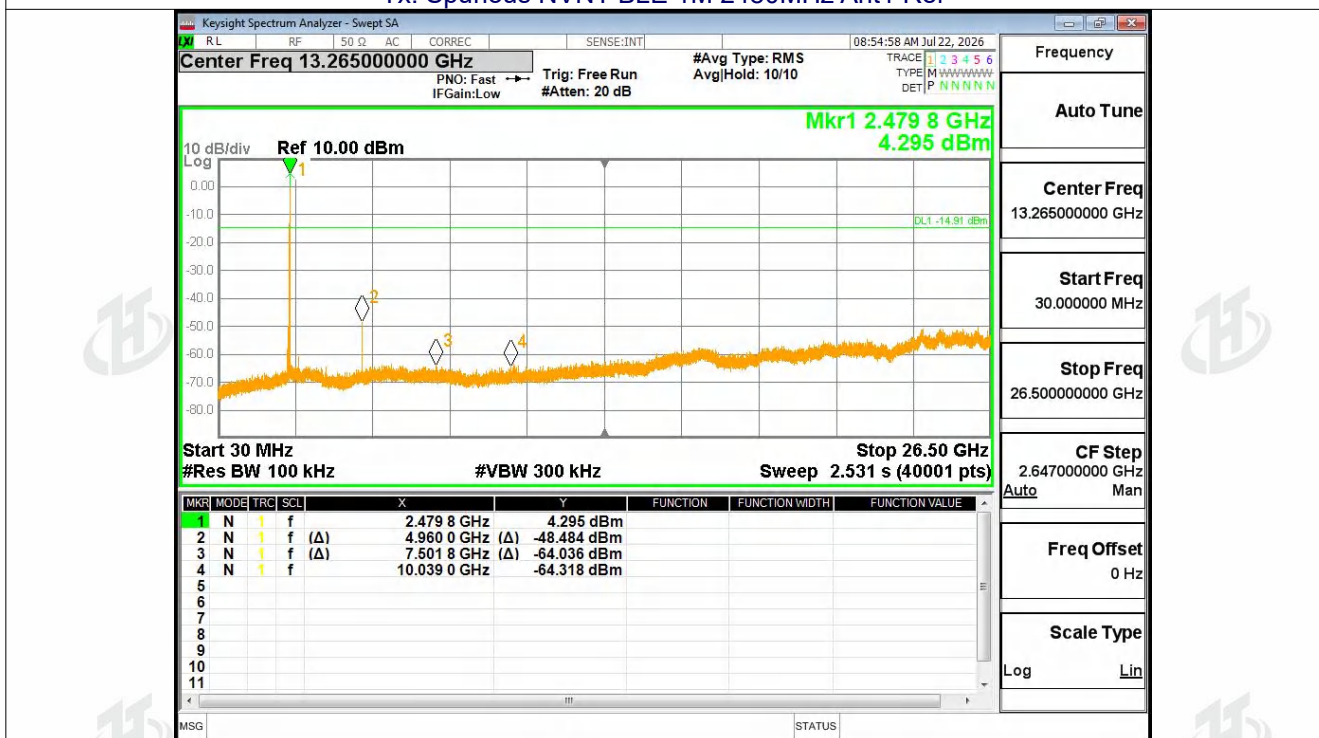
Tx. Spurious NVNT BLE 1M 2480MHz Ant1 Emission
