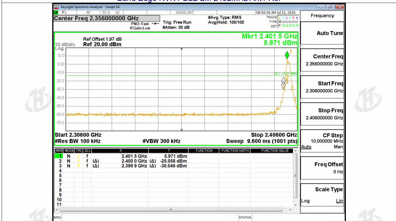
Band Edge NVNT BLE 2M 2402MHz Ant1 Emission
