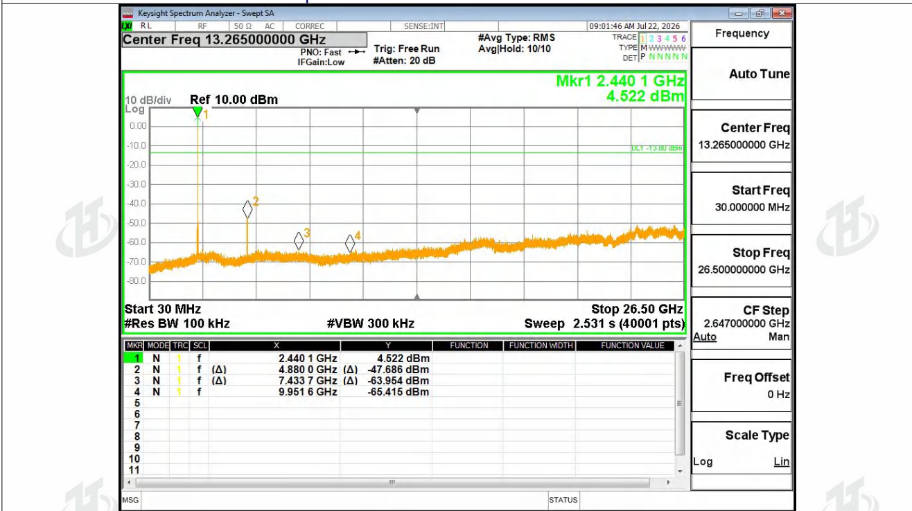
Tx. Spurious NVNT BLE 2M 2440MHz Ant1 Emission
