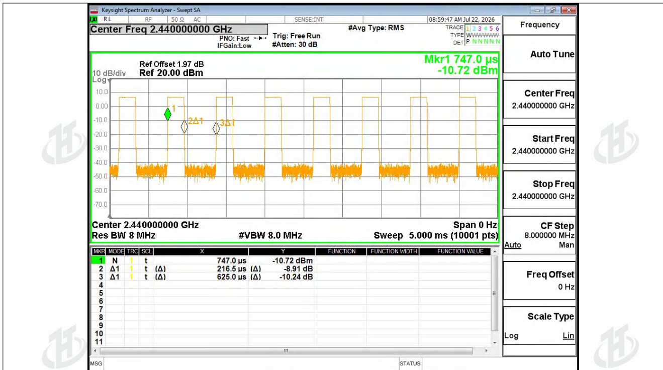
Duty Cycle NVNT BLE 2M 2440MHz Ant1
