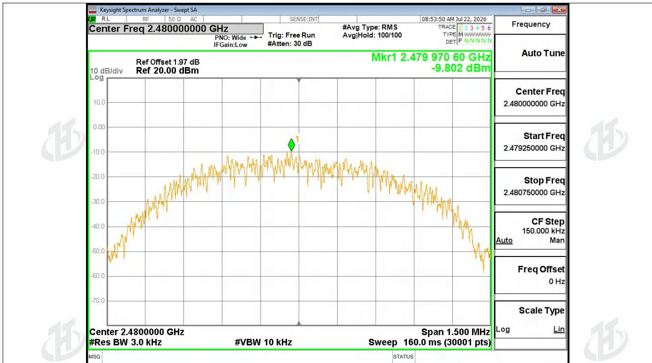
PSD NVNT BLE 1M 2480MHz Ant1
