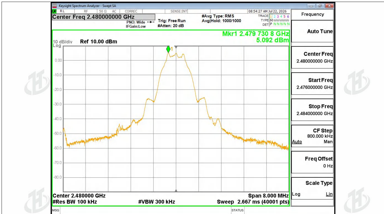
Tx. Spurious NVNT BLE 1M 2480MHz Ant1 Ref
