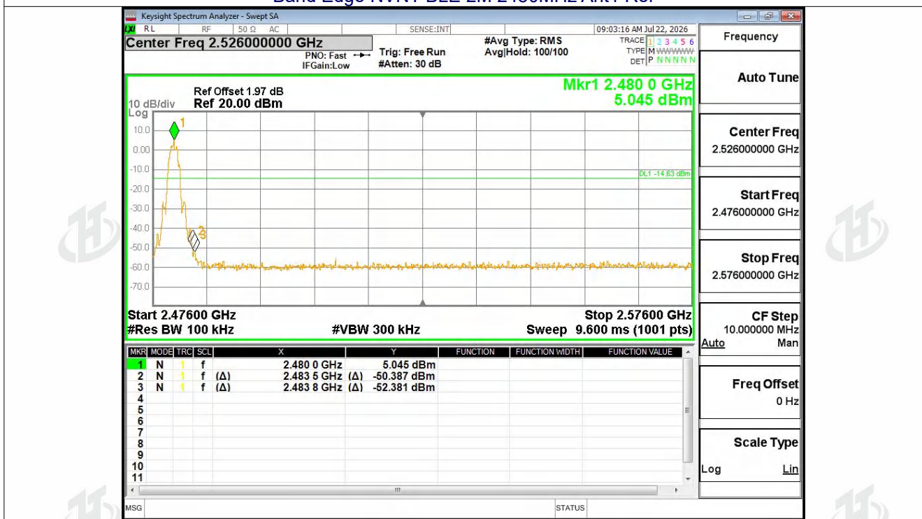
Band Edge NVNT BLE 2M 2480MHz Ant1 Emission
