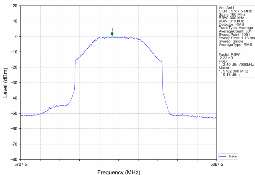
80M_MCH_5787.5MHz_MIMO_NTNV
