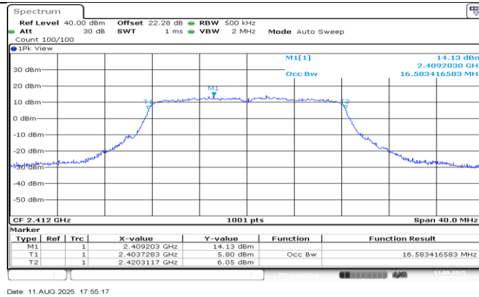
11G-MIMO_Ant1_2412
