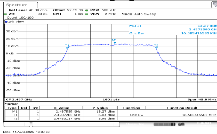
11G-MIMO_Ant1_2437
