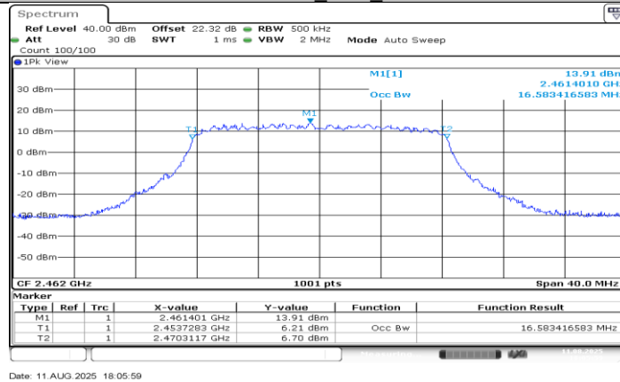
11G-MIMO_Ant2_2462
