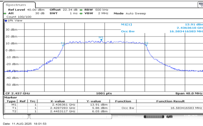
11G-MIMO_Ant2_2437
