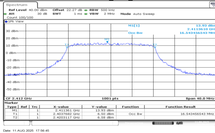
11G-MIMO_Ant2_2412
