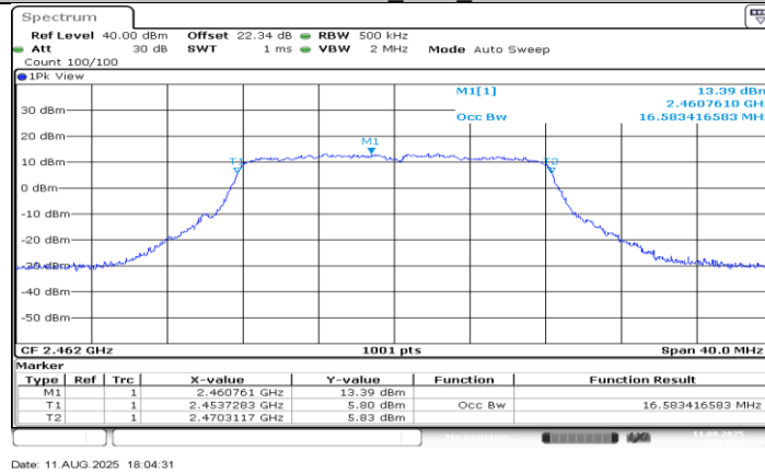
11G-MIMO_Ant1_2462
