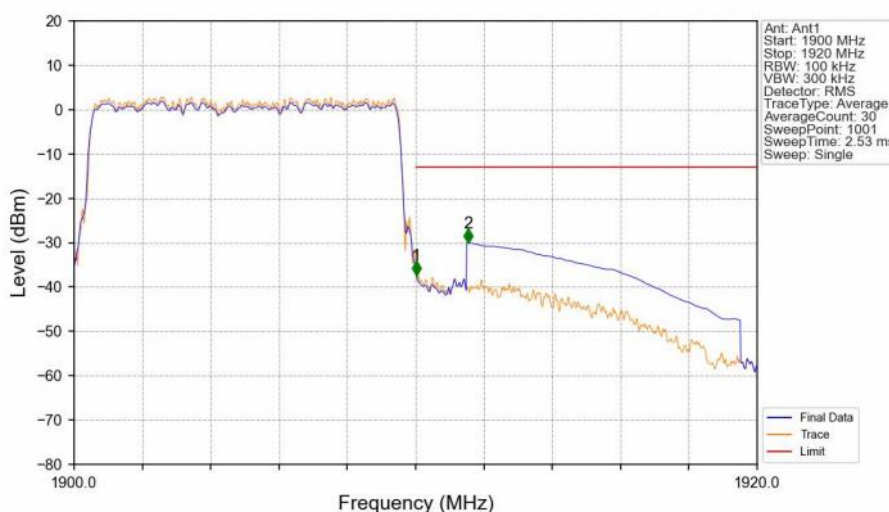
Band2_10MHz_16QAM_HCH_1905MHz_RB_50_0_NTNV
