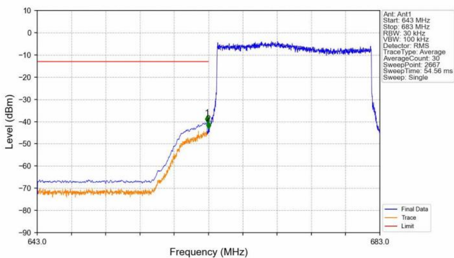
Band71_20MHz_16QAM_LCH_673MHz_RB_100_0_NTNV
