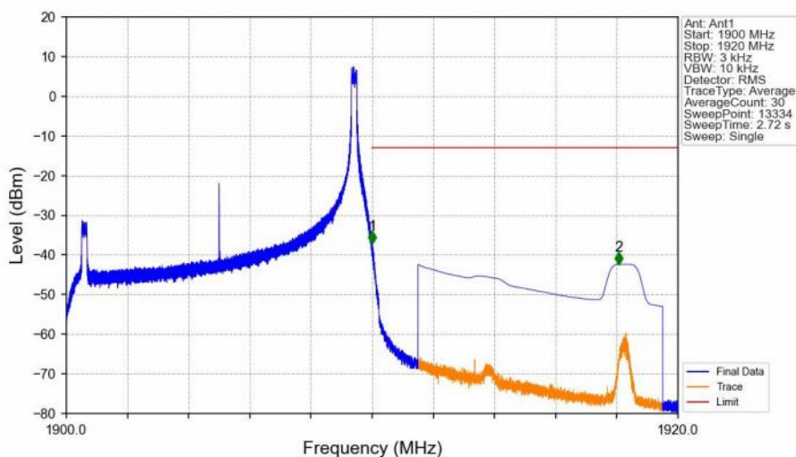
Band2_10MHz_16QAM_HCH_1905MHz_RB_1_49 NTN
