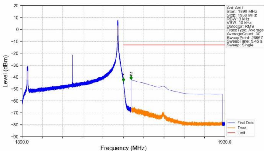
Band2_20MHz_16QAM_HCH_1900MHz_RB_1_99_NTNV
