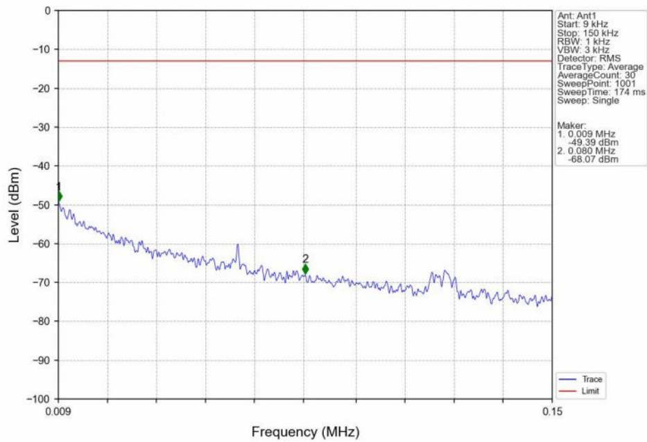
Band2_10MHz_16QAM_MCH_1880MHz_RB_1_0_NTNV
