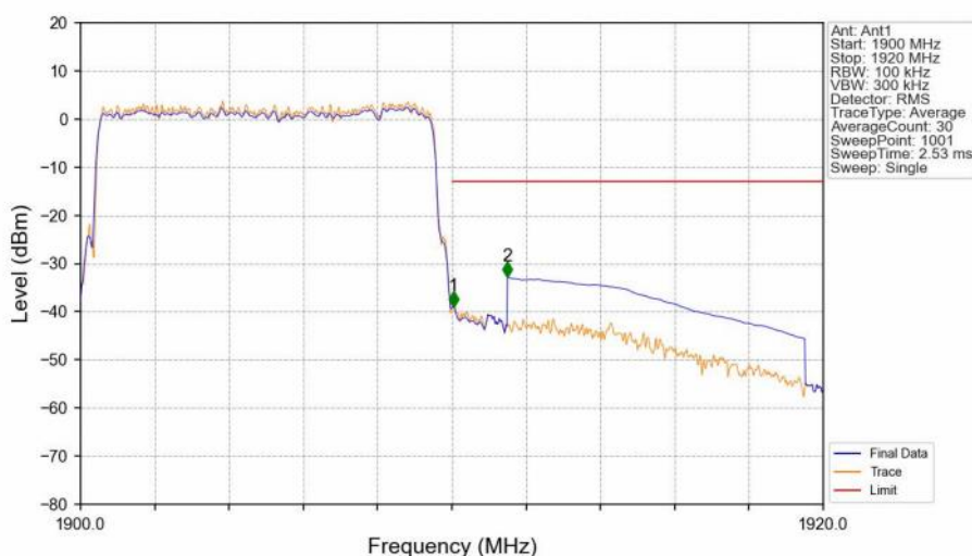
Band2_10MHz_16QAM_HCH_1905MHz_RB_50_0 NTN
