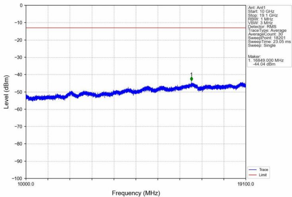
Band2_15MHz_QPSK_LCH_1857.5MHz_RB_1_0_NTNV
