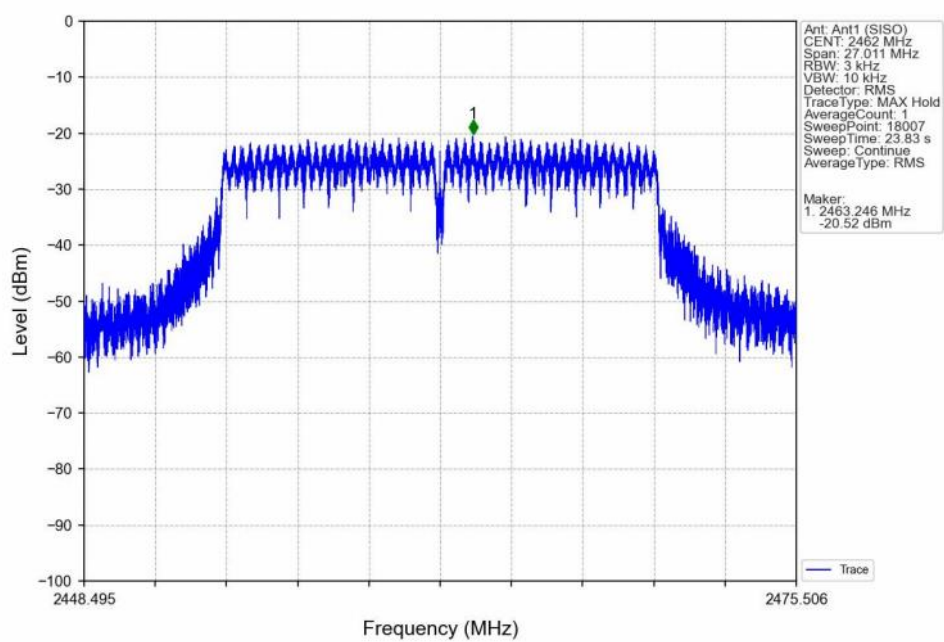
802.11g_HCH_2462MHz_Ant1 (SISO)_NTNV
