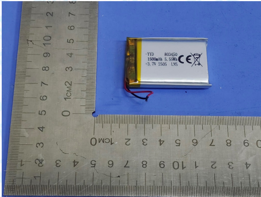
Photo 12 Battery parameters
