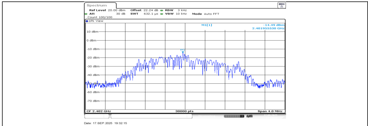
BLE_2M_Ant1_2402
