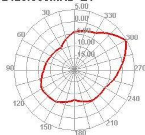
2420.000MHz E1
