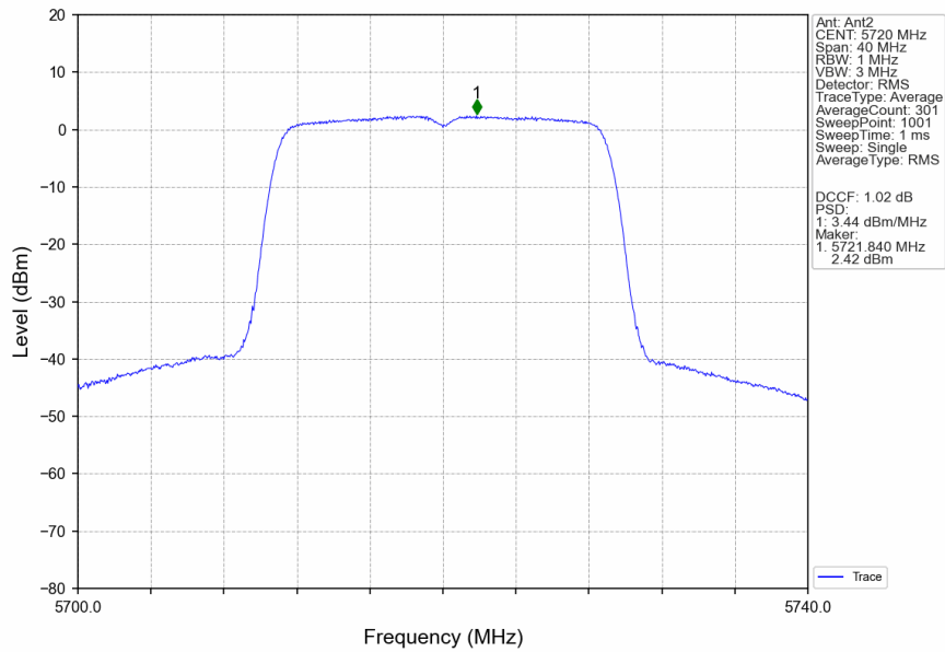
802.11n(HT20)_HCH_5720MHz_MIMO_NTNV
