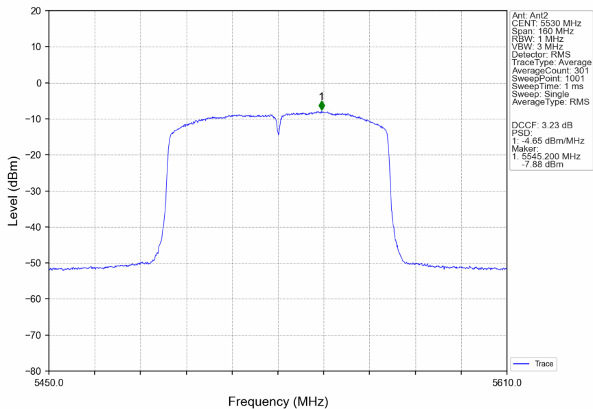
802.11ac(VHT80)_LCH_5530MHz_Ant2_NTNV
