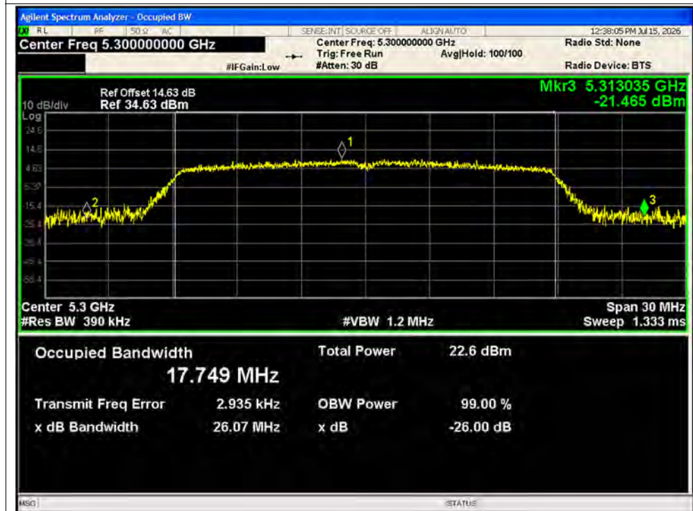
-26dB Bandwidth NVNT ac20 5300MHz Ant1
