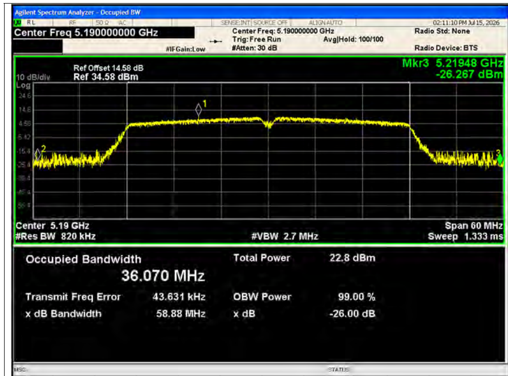
-26dB Bandwidth NVNT n40 5190MHz Ant1
