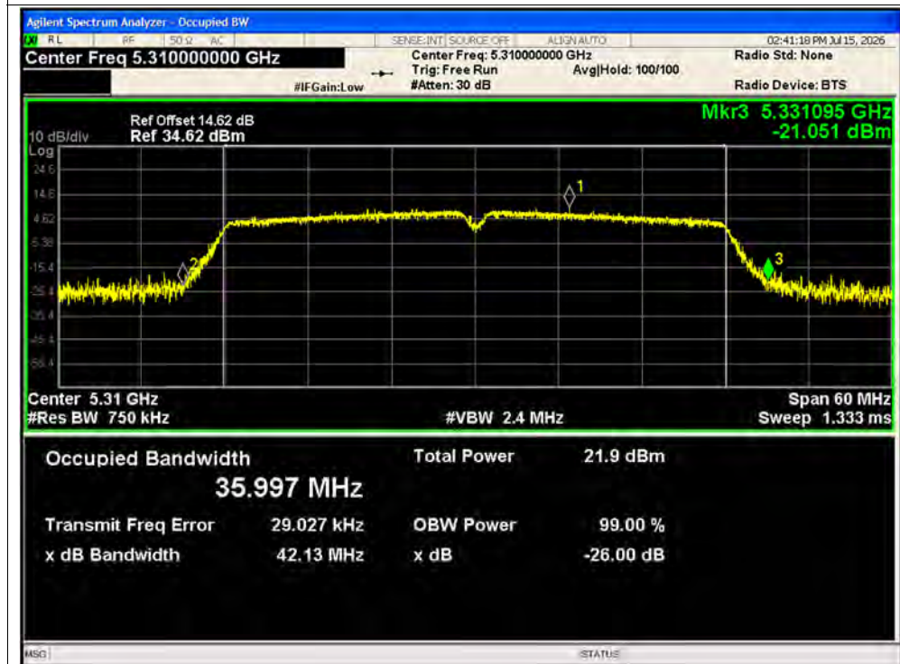
-26dB Bandwidth NVNT ac40 5310MHz Ant1
