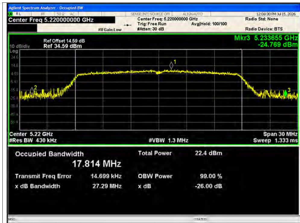
-26dB Bandwidth NVNT n20 5220MHz Ant1
