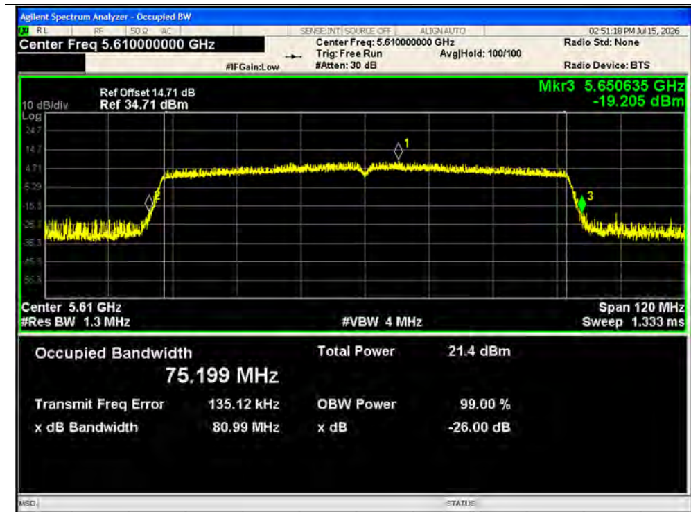
-26dB Bandwidth NVNT ac80 5610MHz Ant1
