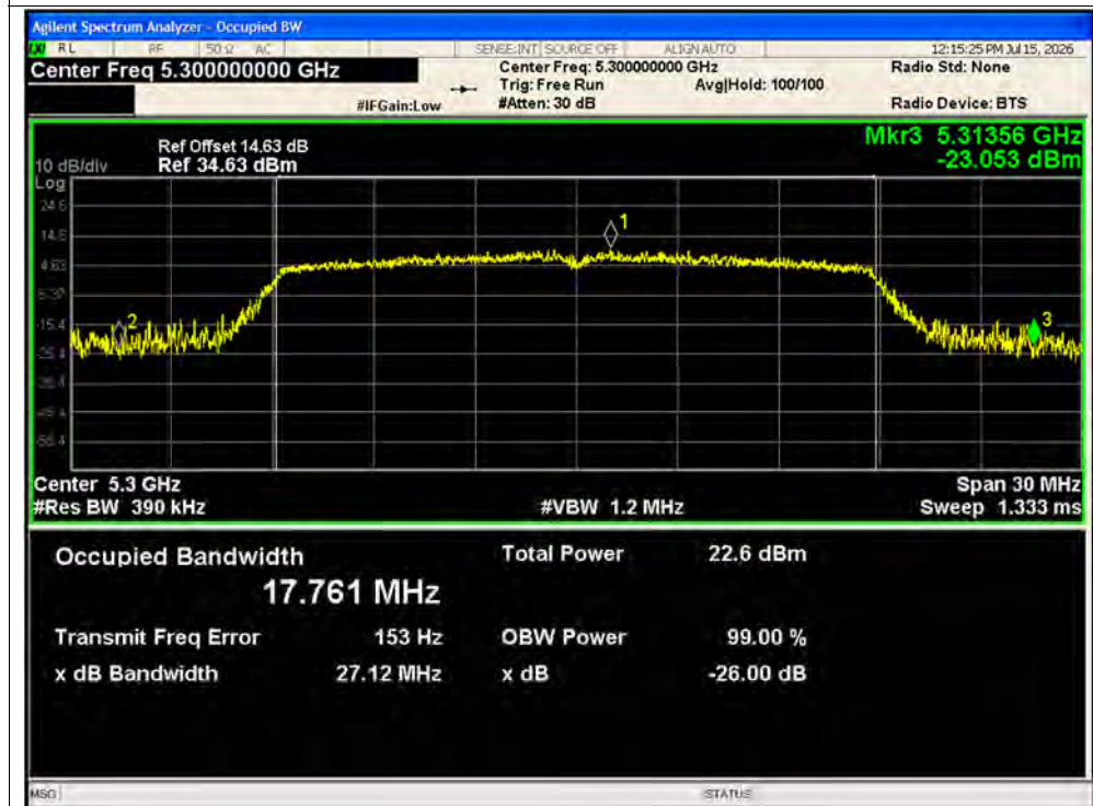
-26dB Bandwidth NVNT n20 5300MHz Ant1
