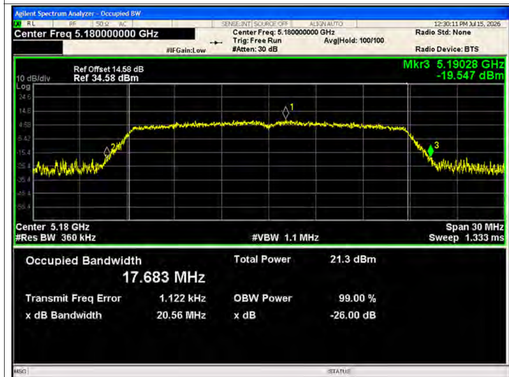
-26dB Bandwidth NVNT ac20 5180MHz Ant1
