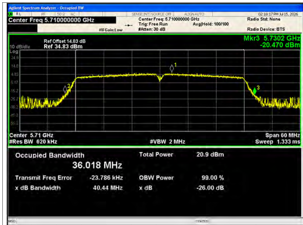
-26dB Bandwidth NVNT n40 5710MHz Ant1
