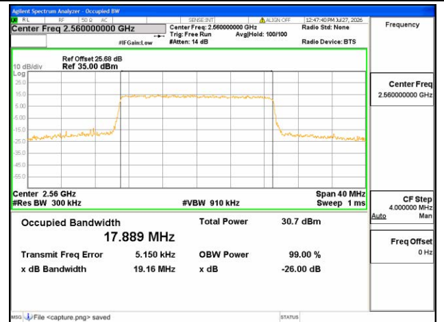
B7 / 20MHz / QPSK/ High CH
