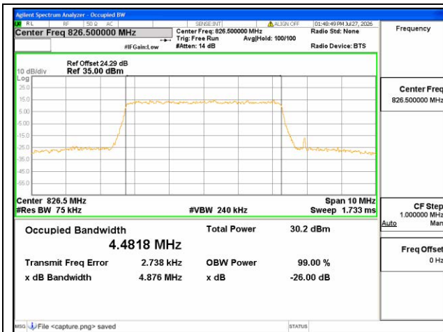
B26 Part22 / 5MHz / QPSK/ Low CH
