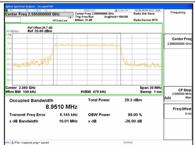
B38 / 10MHz / 16QAM / Mid CH
