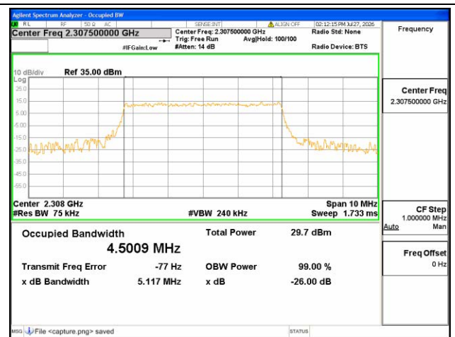
B40-1 / 5MHz / 16QAM / Low CH
