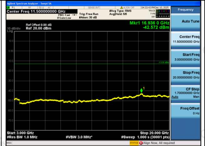
GPRS1900-661-0-3000~20000MHz-PASS
