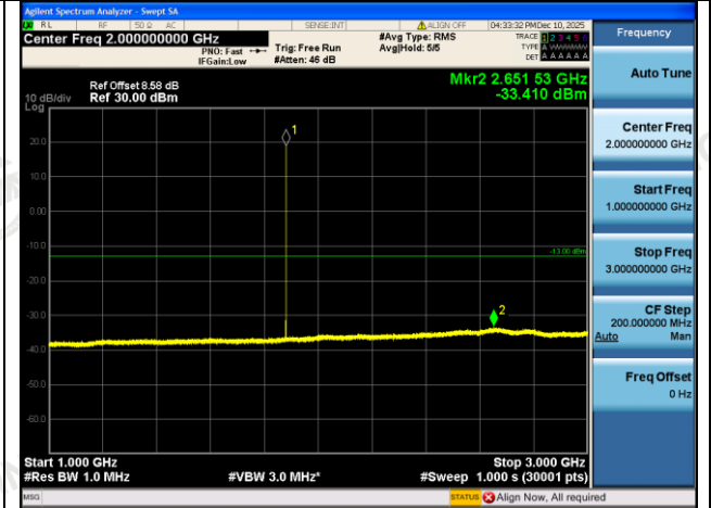
GPRS1900-661-0-1000~3000MHz-PASS
