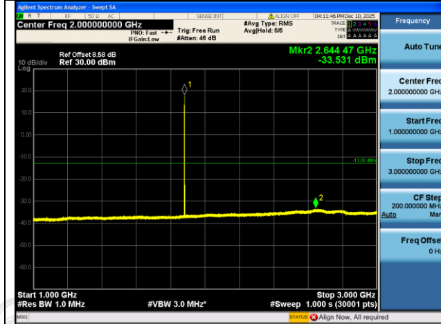
GSM1900-661-0-1000~3000MHz-PASS
