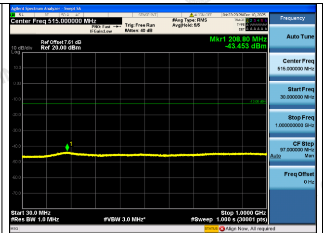
GPRS1900-661-0-30~1000MHz-PASS
