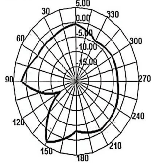
2450.000MHz E2
