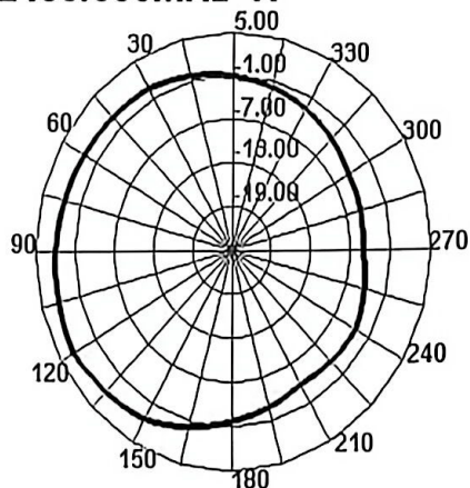
2400.000MHz H
