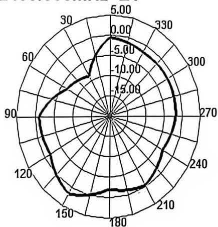
2400.000MHz E1
