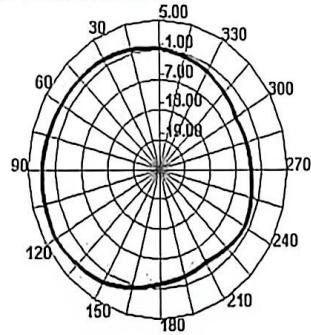
2450.000MHz H
