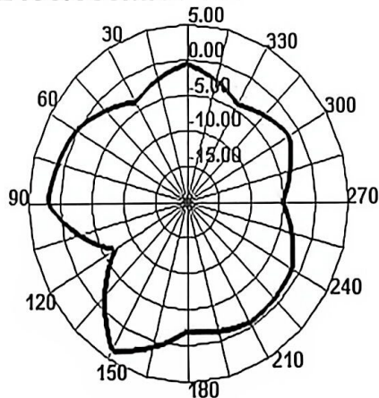
2400.000MHz E2
