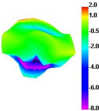
5150.000MHz E1
