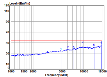
BLE_2M_TX_CH_19_Vertical-Avg
