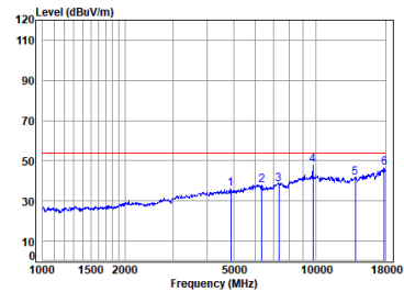
BLE_2M_TX_CH_19_Horizontal-Avg
