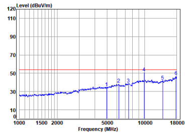
BLE_2M_TX_CH_39_Horizontal-Avg
