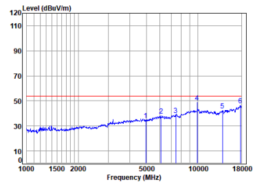
BLE_2M_TX_CH_39_Vertical-Avg
