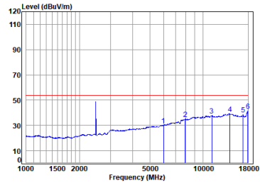
BLE_2M_TX_CH_38_Vertical-Avg
