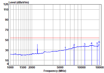
BLE_2M_TX_CH_01_Horizontal-Avg
