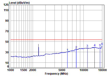
BLE_2M_TX_CH_01_Vertical-Avg
