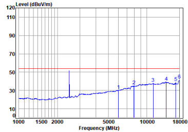
BLE_2M_TX_CH_38_Horizontal-Avg
